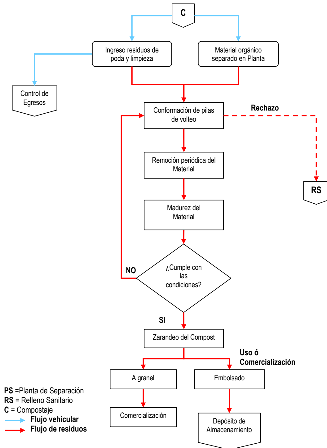
Figura 18: Flujograma Sector de Compostaje
