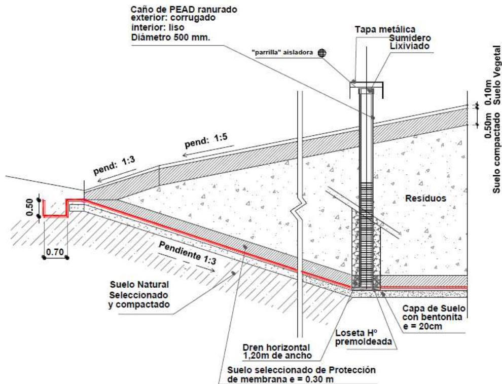
Figura 9: Detalle sumidero de extracción de lixiviados
