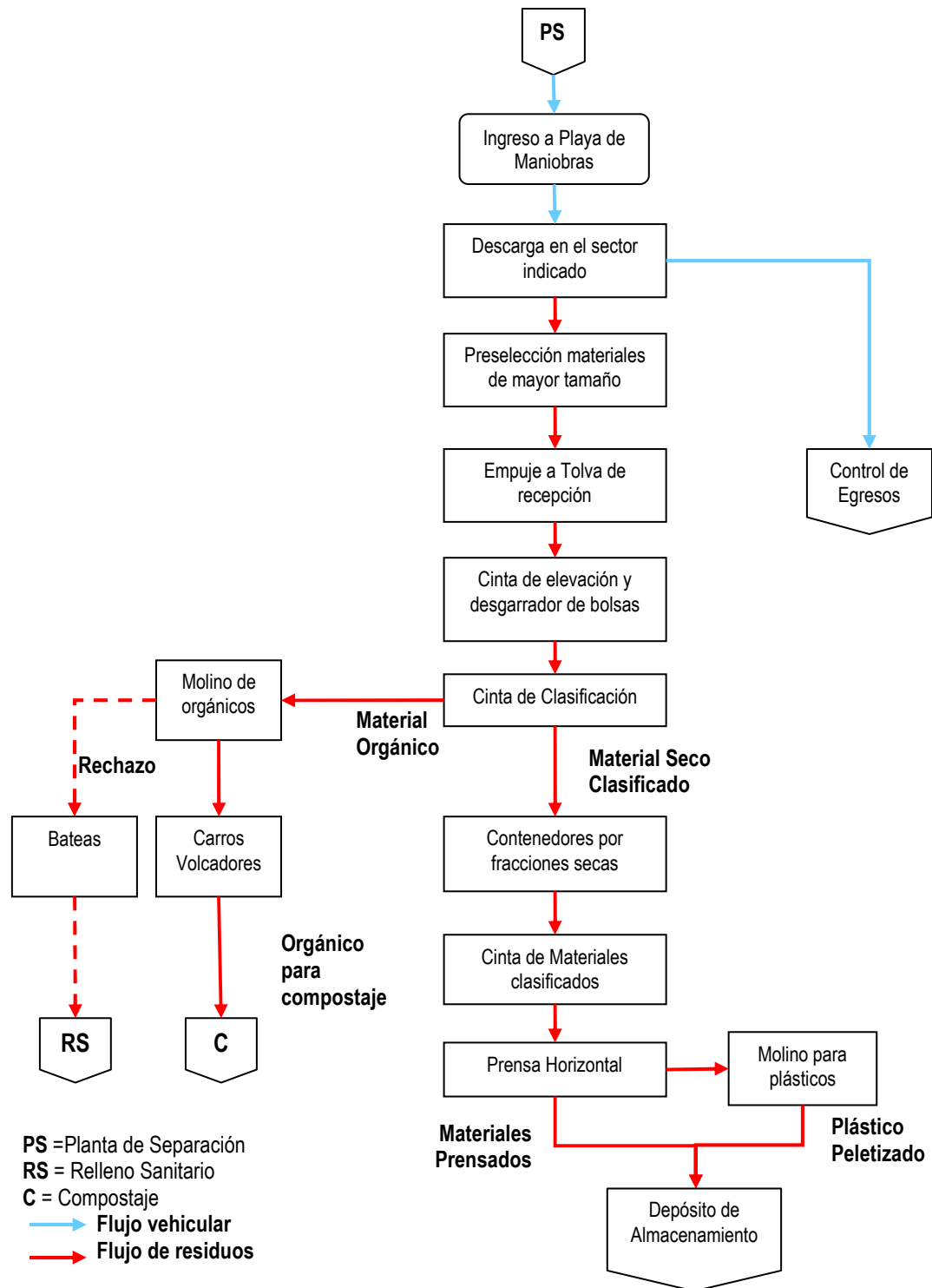
Figura 17: Flujograma Planta de Separación
