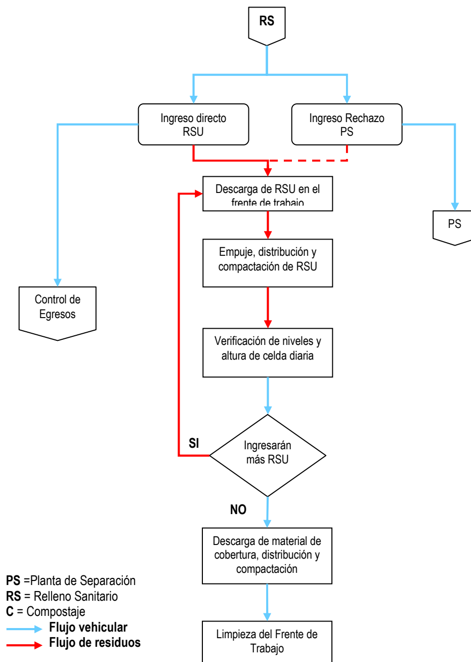
Figura 19: Flujograma Relleno Sanitario
