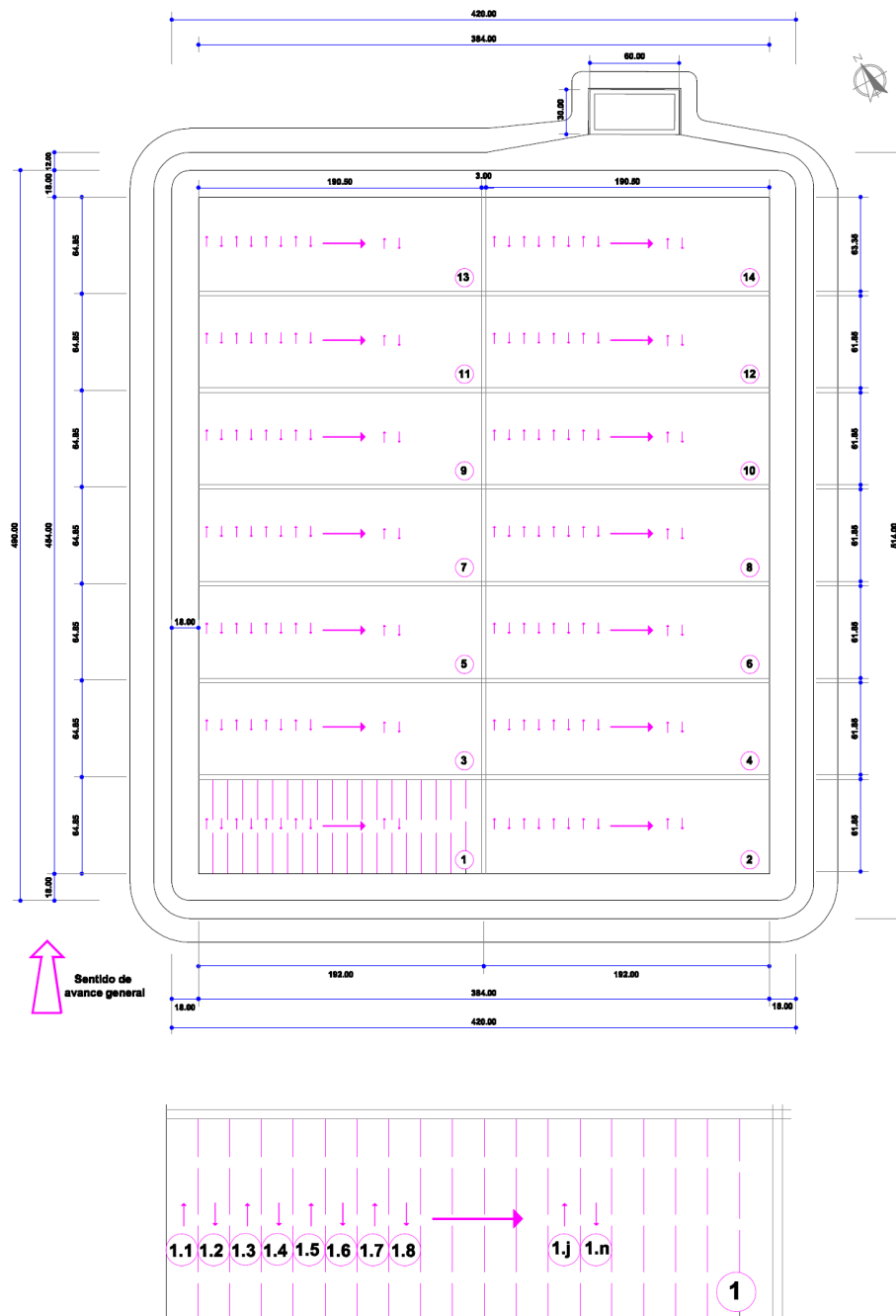
Figura 15: Secuencia Constructiva del Módulo 1
