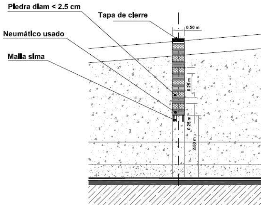
Figura 11: Corte tubos de reinyección de líquidos lixiviados
