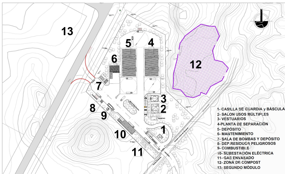
Figura 14: Planimetría General del Sector de Edificios Complementarios
