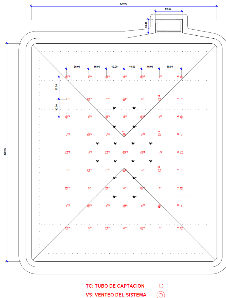
Figura 12: Distribución de las chimeneas de venteo de Biogás
