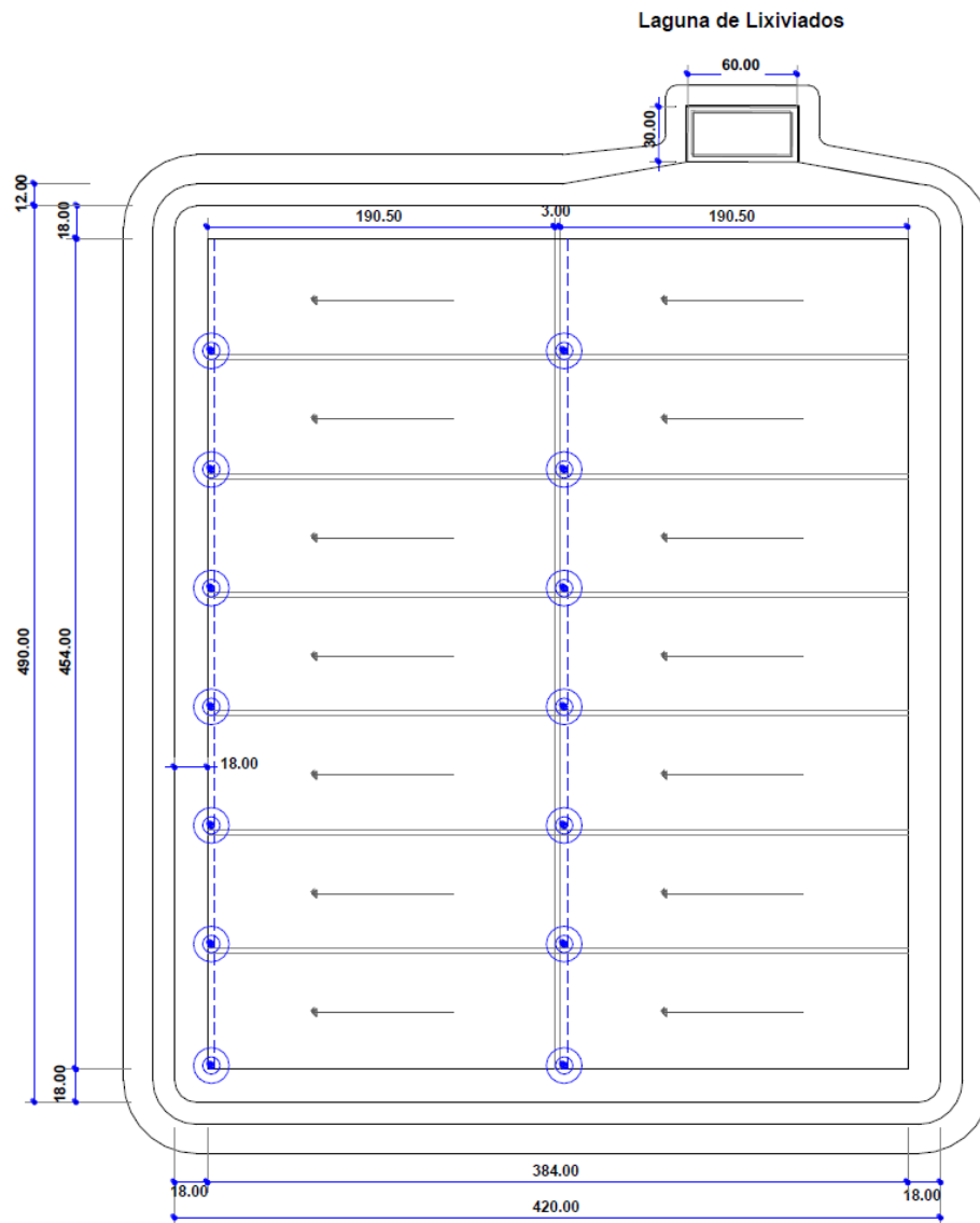
Figura 8: Esquema en planta – Distribución de conductos de captación de lixiviados
