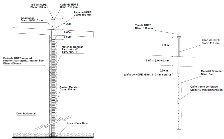
Figura 13: Detalle de las chimeneas de venteo de Biogás
