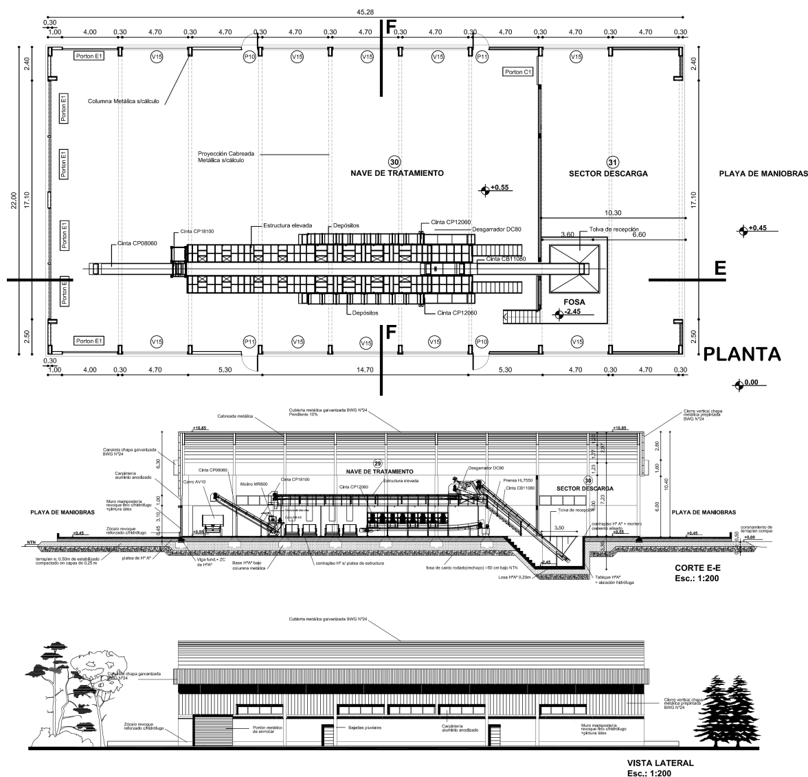
Figura 7: Croquis de Planta, Corte Transversal y Vista Lateral Planta de Separación
