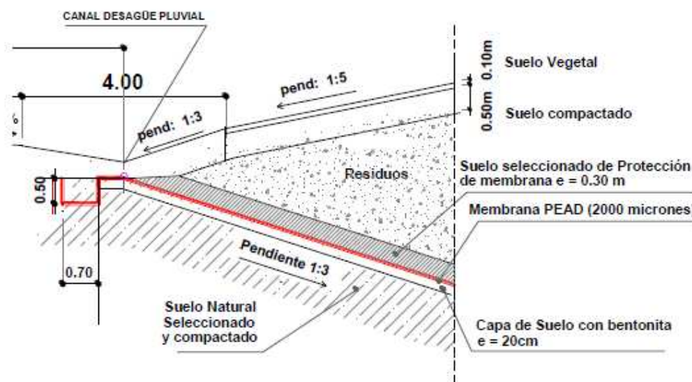
Figura 4: Detalle de impermeabilización y cobertura Módulo
