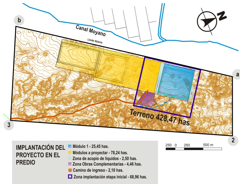
Figura 3: Esquema de Implantación del proyecto
