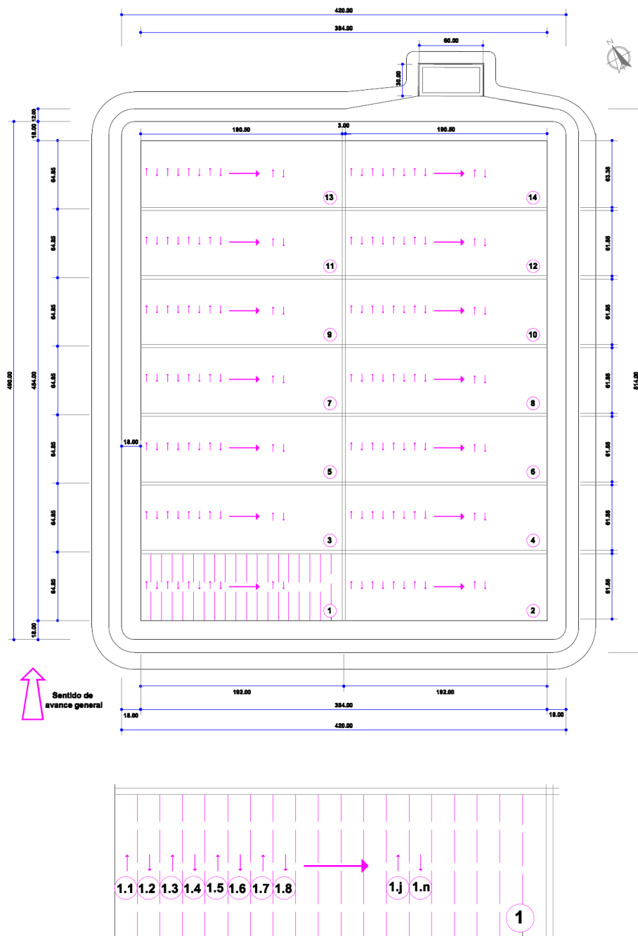
Figura 5: Secuencia Constructiva del Módulo
