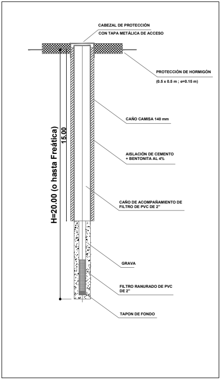
Detalle constructivo de pozo de monitoreo de aguas subterráneas
