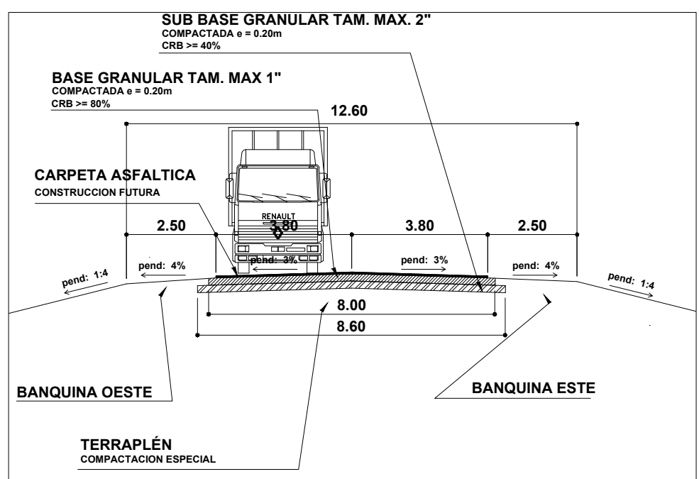
PERFIL TRANSVERSAL DE CAMINO DE ACCESO
