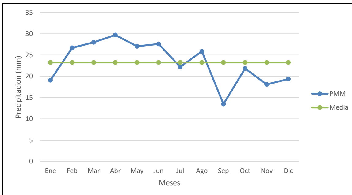
Gráfica 5.5 Precipitación media mensual del período 1993 a 2023
