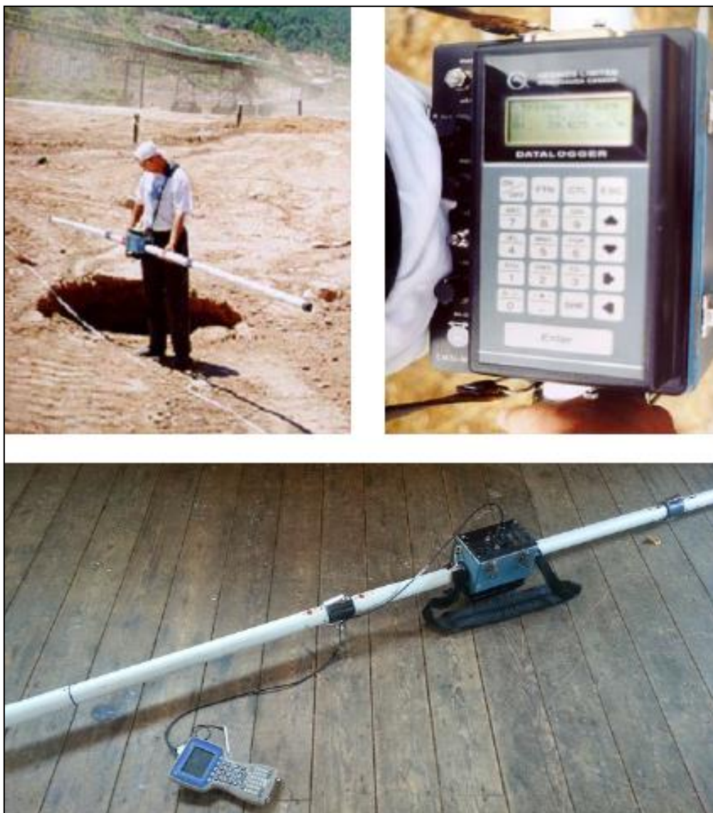
Fotografía 20.2 Vista de los elementos de un sistema electromagnético.
