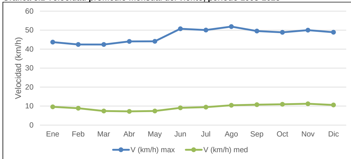
Gráfica 5.1 Velocidad promedio mensual del viento, período 1993-2023
