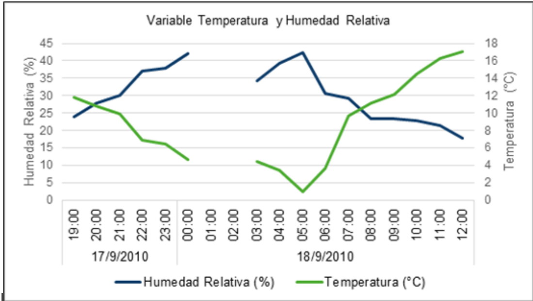
Gráfica 6.7 Variación de la temperatura y humedad relativa durante el periodo de monitoreo. Punto 3: Localidad Bardas Blancas – Escuela Peregrina Cantos.
