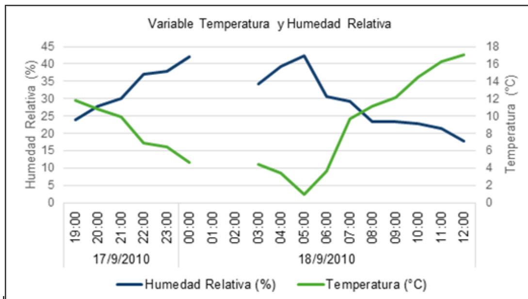
Gráfica 6.14 Variación de la temperatura y humedad relativa durante el periodo de monitoreo. Punto 3: Localidad Bardas Blancas – Escuela Peregrina Cantos.
