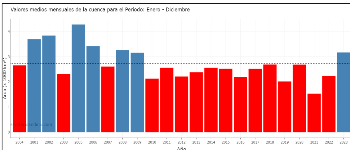
Gráfica 5.14 Valores de superficie promedio mensual cubierta por nieve de la cuenca del río Colorado
