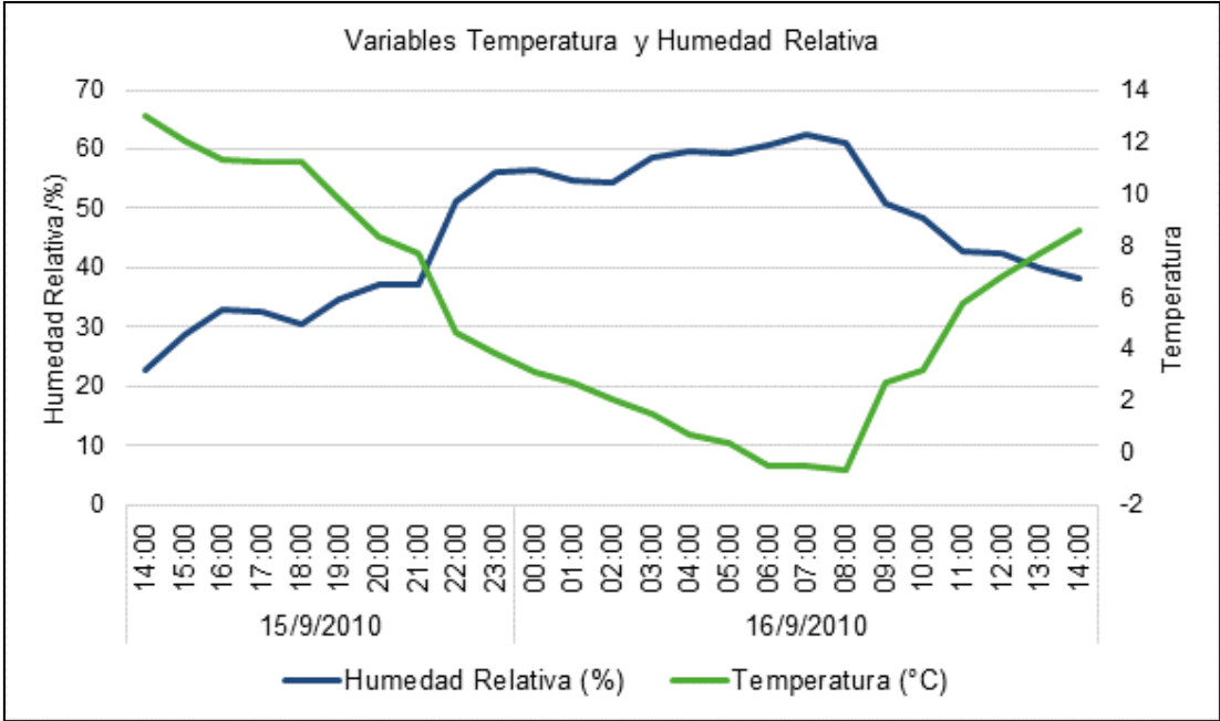
Gráfica 6.7 Variación de la temperatura y humedad relativa durante el período de monitoreo. Punto 2: Zona Industrial Malargüe – Planta de Ecogas
