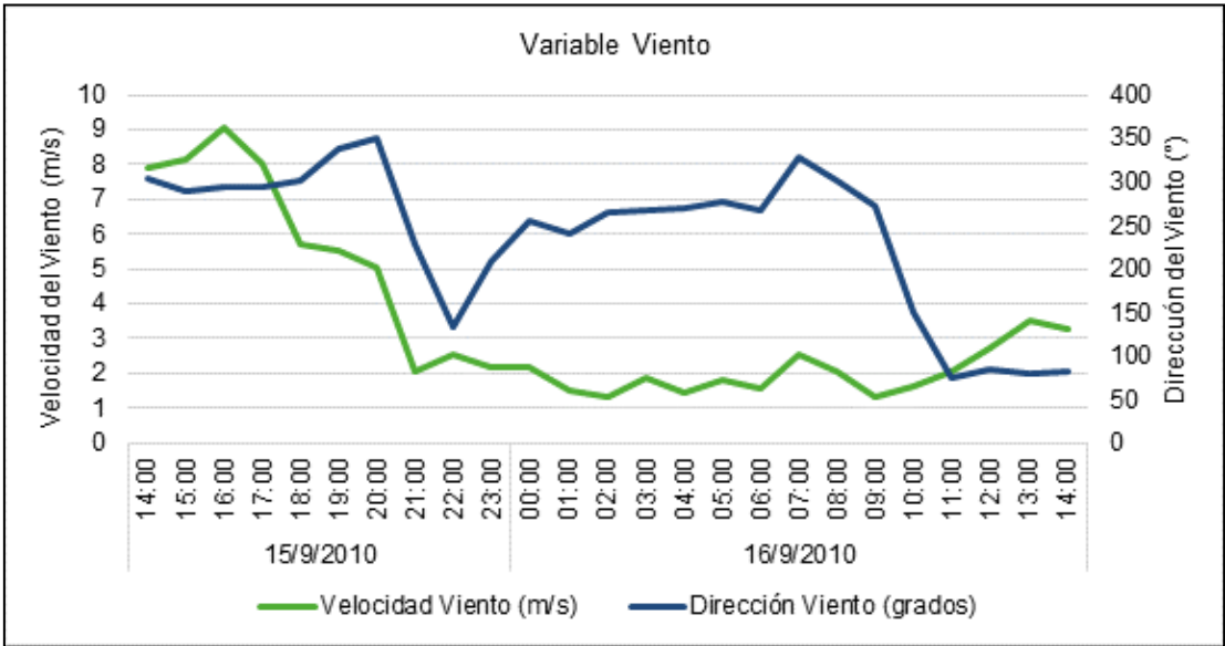
Gráfica 6.6 Variación de la velocidad y dirección del viento durante el período de monitoreo. Punto 2: Zona Industrial Malargüe – Planta de Ecogas
