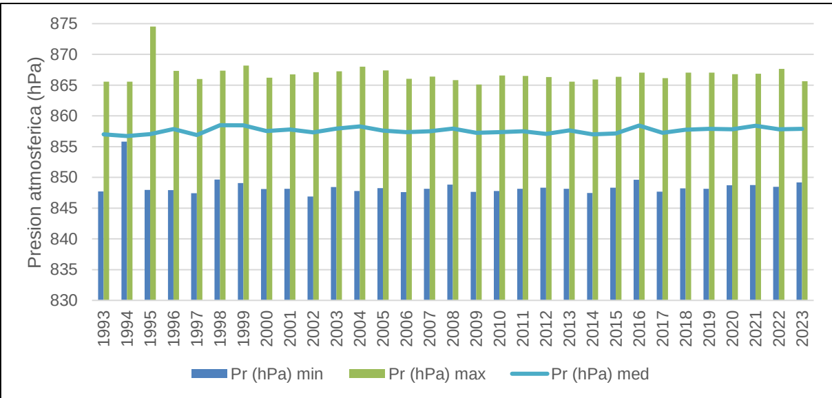
Gráfica 5.10 Presión atmosférica media anual histórica 1993 a 2023
