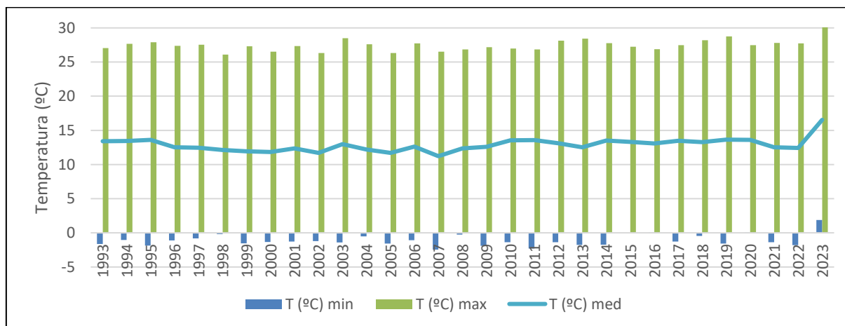
Gráfica 5.12 Temperatura de suelo media anual del período 1993-2023
