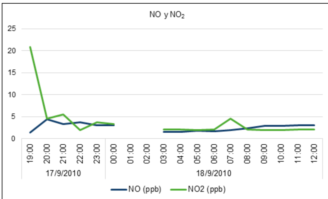
Gráfica 6.10 Variación de la concentración de NO y NO 2 durante el período de monitoreo. Punto 3: Localidad Bardas Blancas – Escuela Peregrina Cantos.
