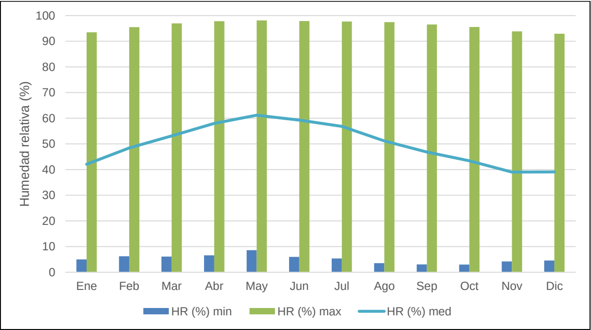
Gráfica 5.7 Humedad relativa del suelo mensual del período 1993 a 2023
