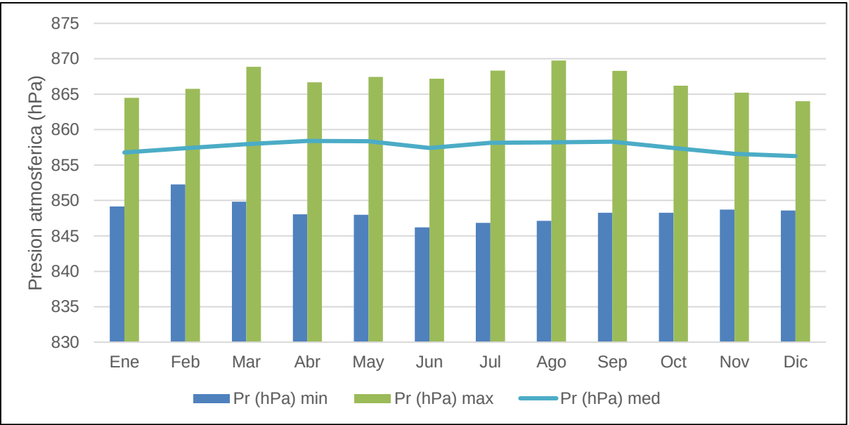
Gráfica 5.9 Presión atmosférica media mensual histórica 1993 a 2023
