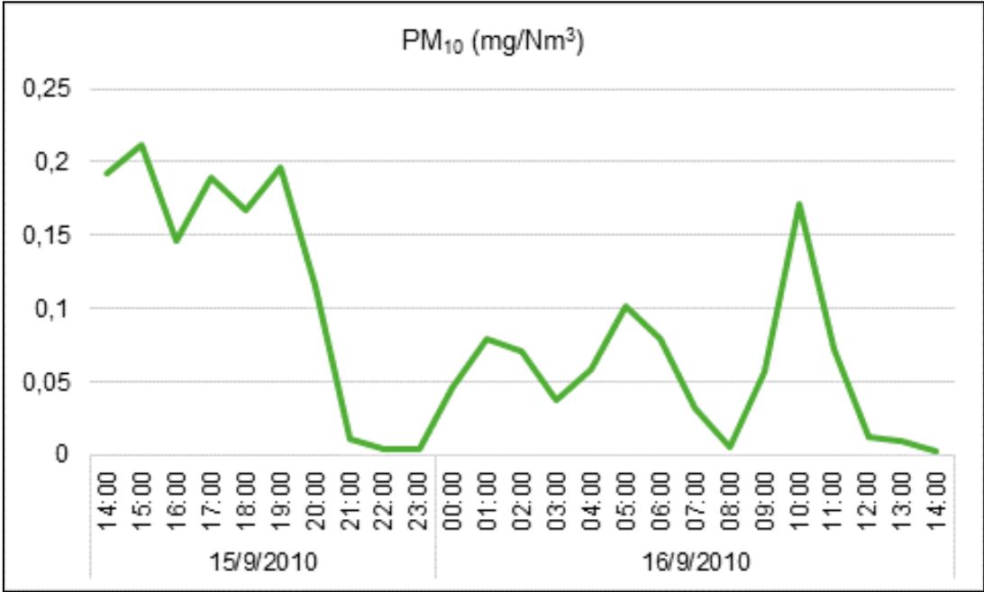
Gráfica 6.1 Variación de la concentración de PM 10 durante el período de monitoreo. Punto 2: Zona Industrial Malargüe – Planta de Ecogas
