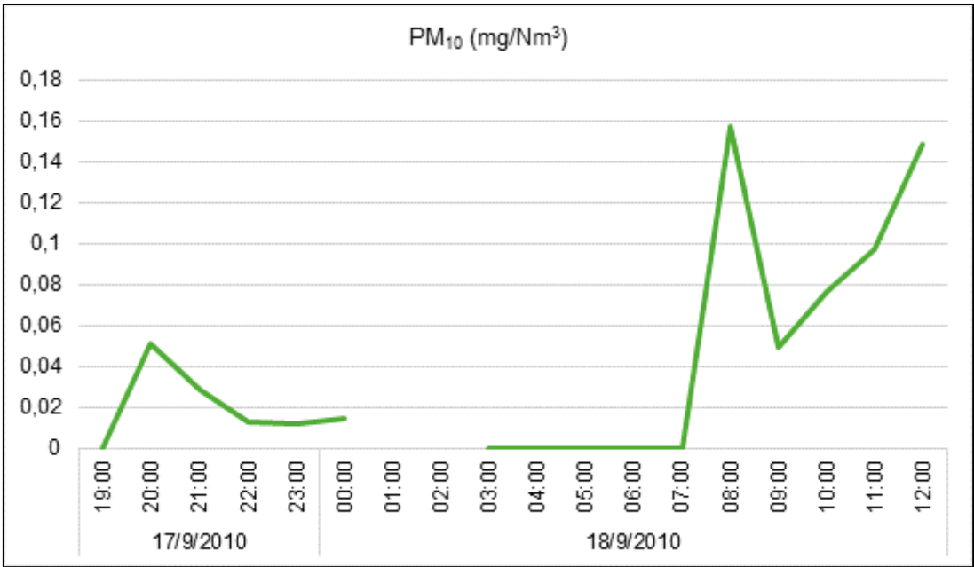
Gráfica 6.8 Variación de la concentración de PM 10 durante el período de monitoreo. Punto 3: Localidad Bardas Blancas – Escuela Peregrina Cantos.
