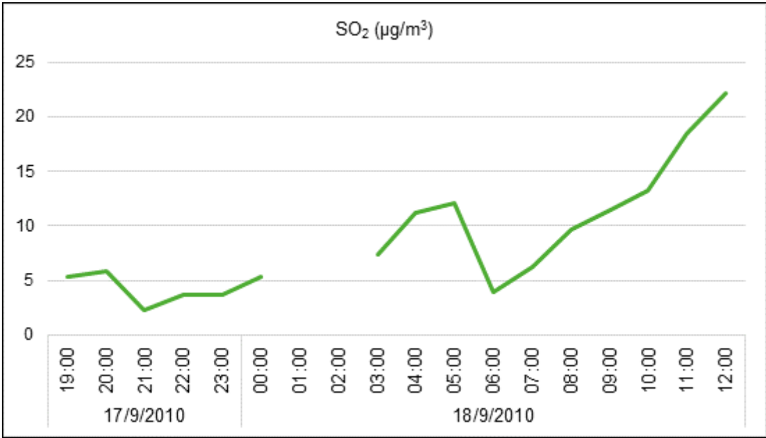
Gráfica 6.9 Variación de la concentración de SO 2 durante el período de monitoreo. Punto 3: Localidad Bardas Blancas – Escuela Peregrina Cantos.
