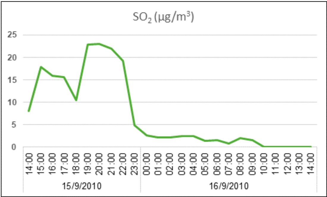
Gráfica 6.2 Variación de la concentración de SO 2 durante el período de monitoreo. Punto 2: Zona Industrial Malargüe – Planta de Ecogas
