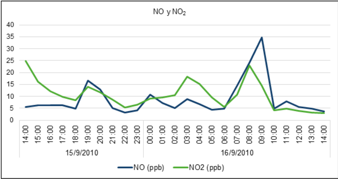
Gráfica 6.3 Variación de la concentración de NO y NO 2 durante el período de monitoreo. Punto 2: Zona Industrial Malargüe – Planta de Ecogas
