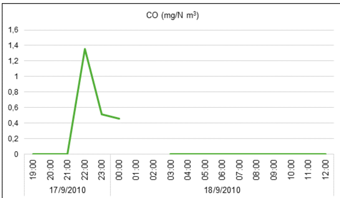
Gráfica 6.11 Variación de la concentración de CO durante el período de monitoreo. Punto 3: Localidad Bardas Blancas – Escuela Peregrina Cantos.
