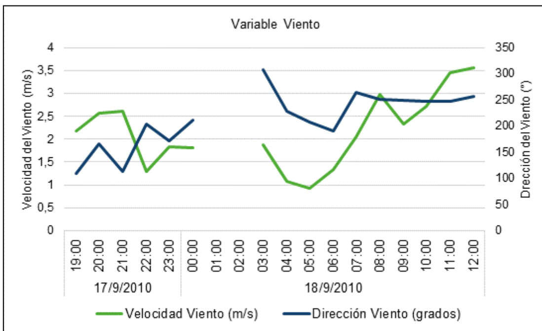
Gráfica 6.13 Variación de la velocidad y dirección del viento durante el periodo de monitoreo. Punto 3: Localidad Bardas Blancas – Escuela Peregrina Cantos.
