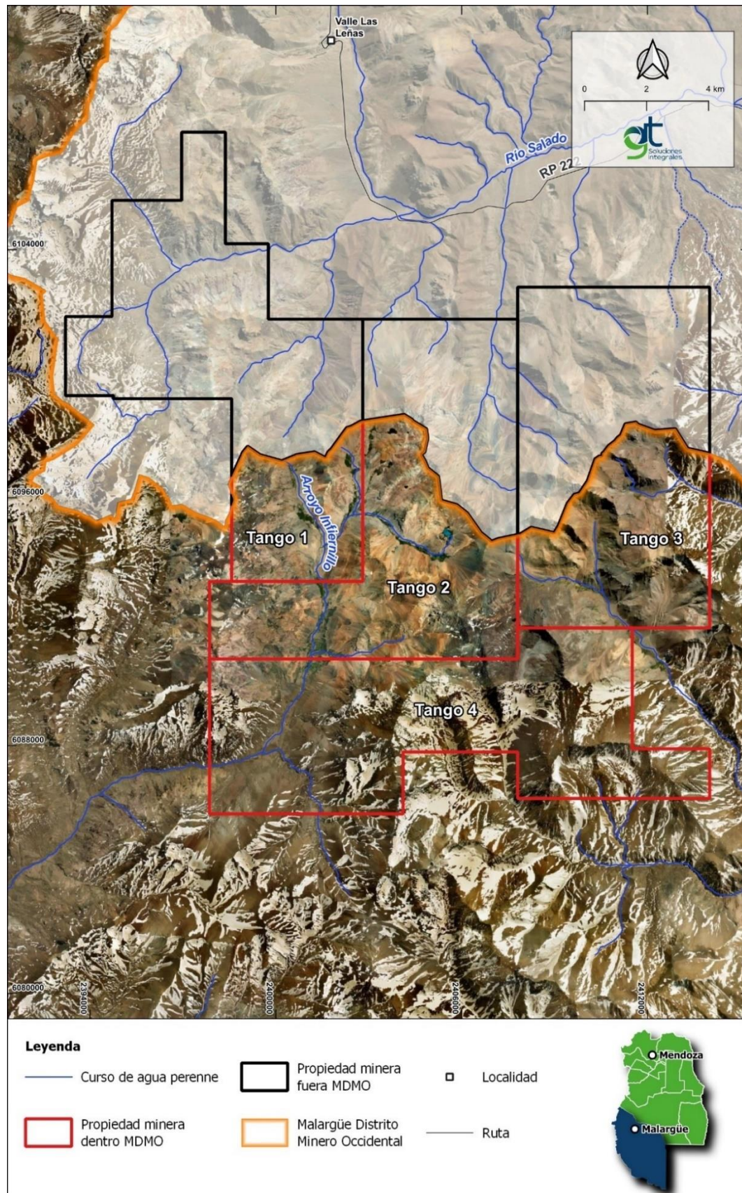
Mapa 7.1 Cursos y cuerpos de agua presentes en el área de Proyecto Tango.
