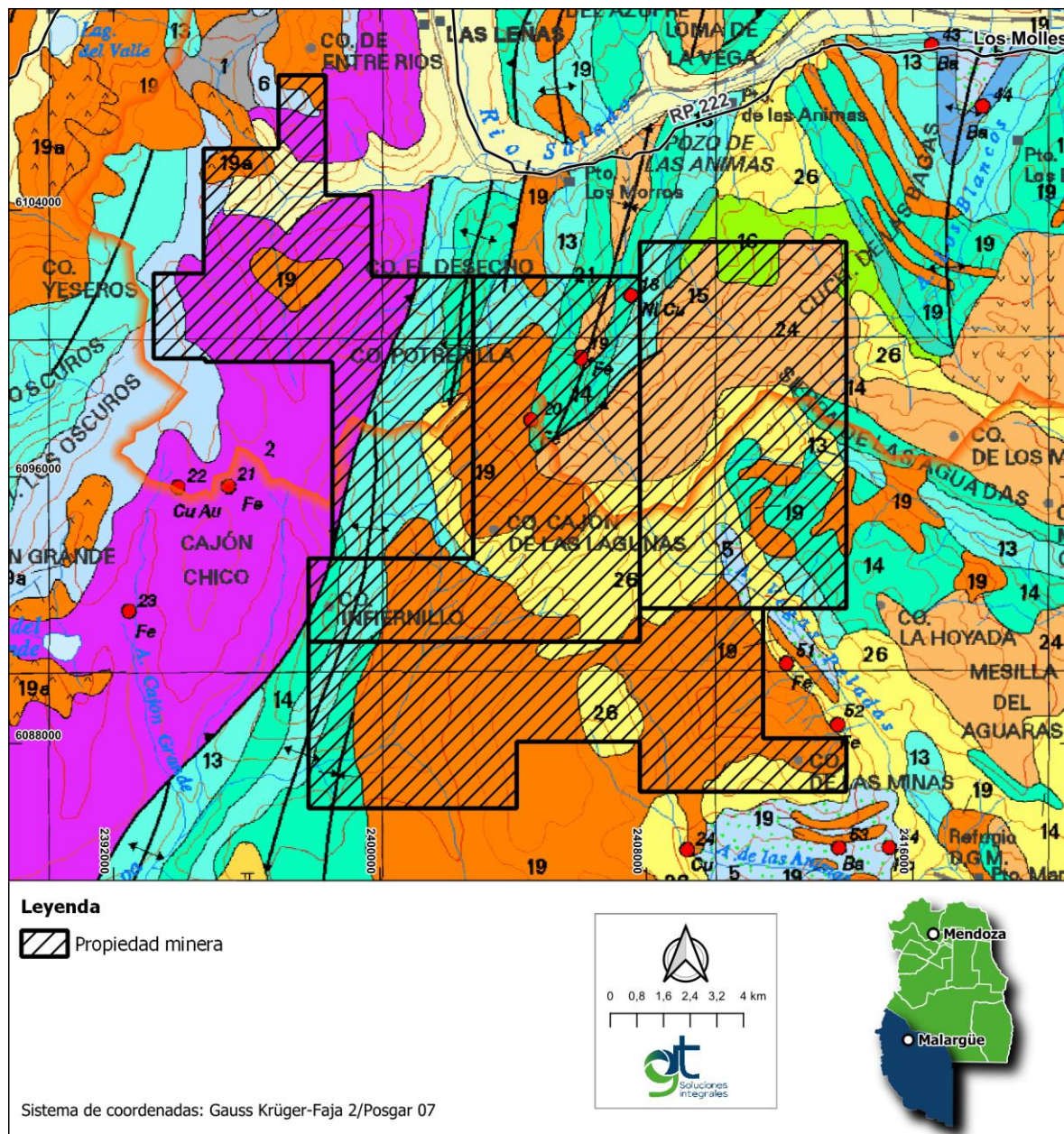
Mapa 3.1 Unidades geológicas aflorantes del área de Proyecto Tango
