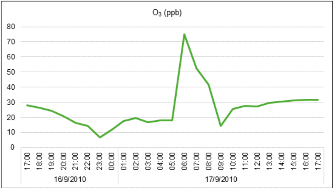
Gráfica 6.5 Variación de la concentración de O 3 durante el periodo de monitoreo. Punto 1: Centro de Malargüe – Predio de Vialidad
