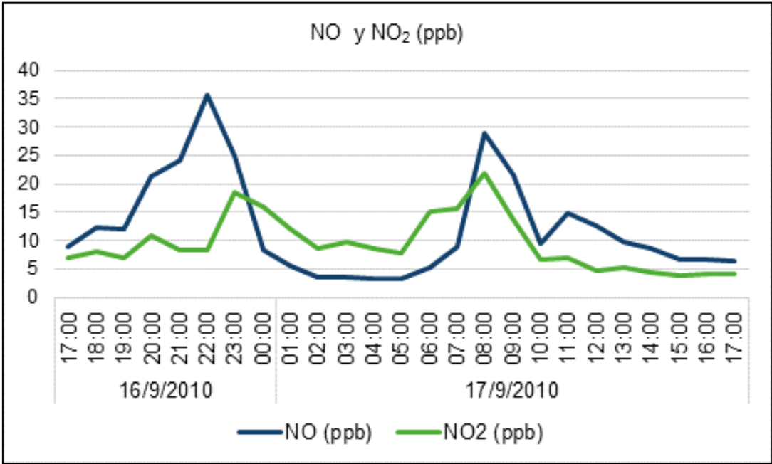
Gráfica 6.3 Variación de la concentración de NO y NO 2 durante el periodo de monitoreo. Punto 1: Centro de Malargüe – Predio de Vialidad
