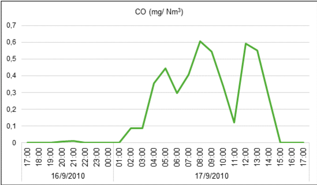
Gráfica 6.4 Variación de la concentración de CO durante el periodo de monitoreo. Punto 1: Centro de Malargüe – Predio de Vialidad
