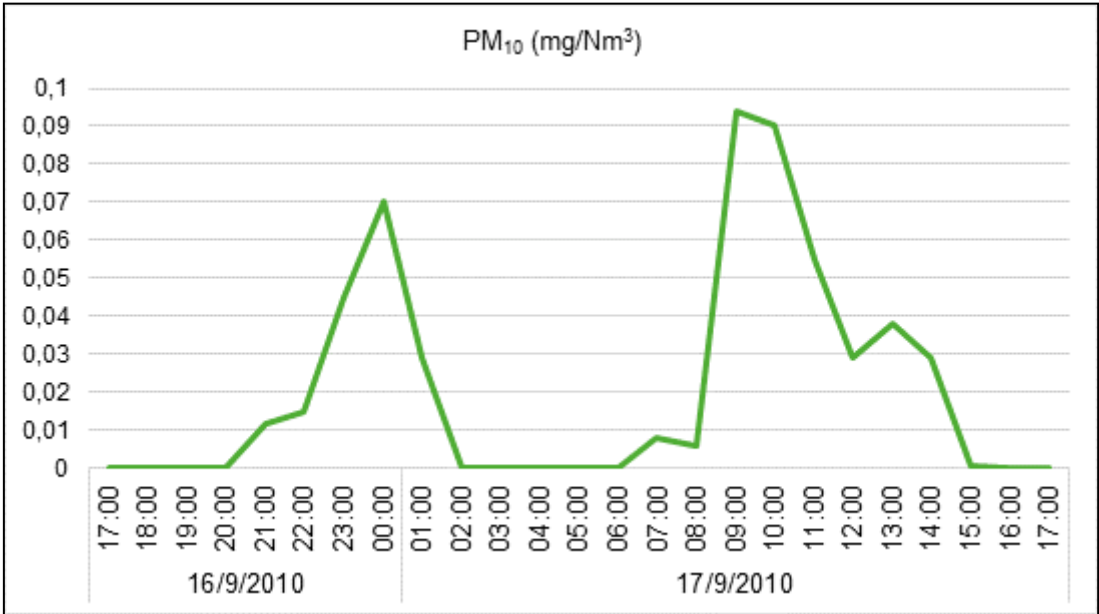
Gráfica 6.1 Variación de la concentración de PM 10 durante el periodo de monitoreo. Punto 1: Centro de Malargüe – Predio de Vialidad
