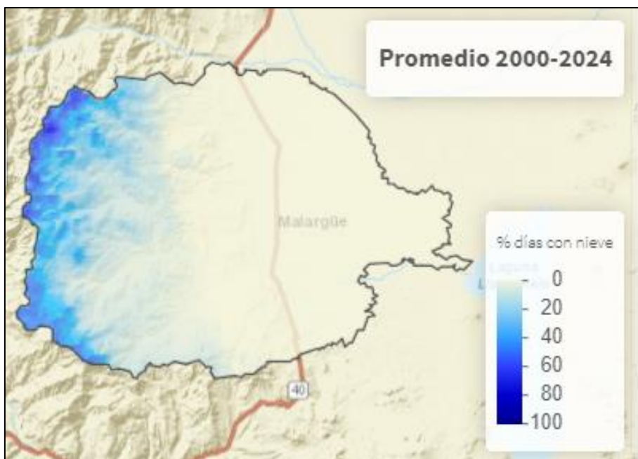
Figura 5.2 Porcentaje de días con nieve en la Cuenca del Río Malargüe
