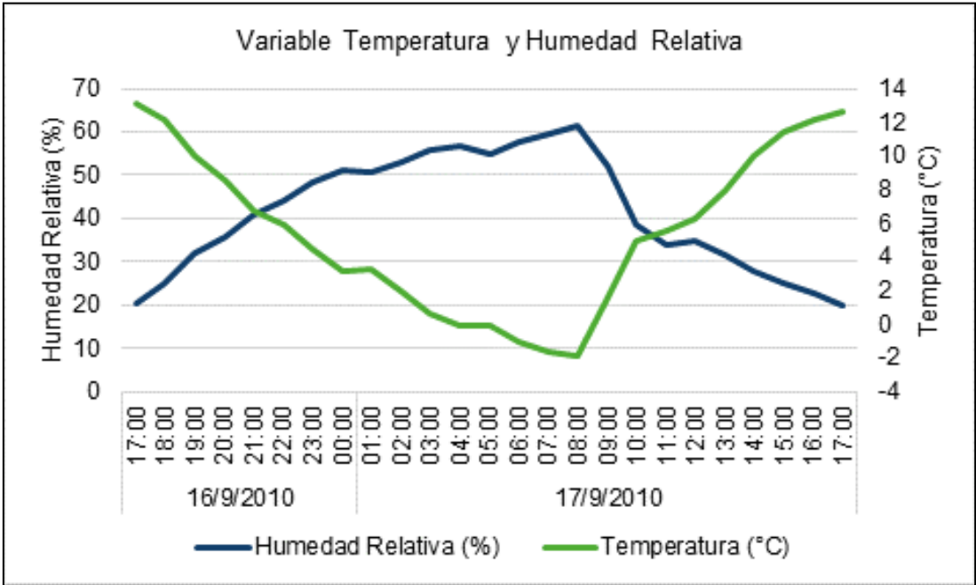
Gráfica 6.7 Variación de la temperatura y humedad relativa durante el periodo de monitoreo. Punto 1: Centro de Malargüe – Predio de Vialidad
