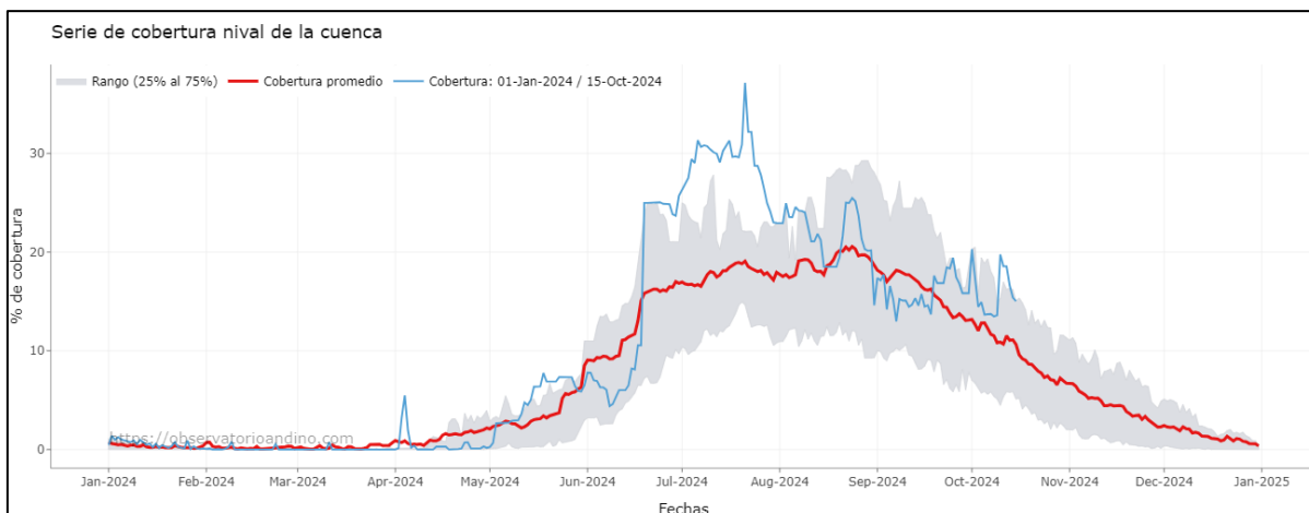
Gráfica 5.15 Coberturas de nieve en la cuenca del Río Malargüe
