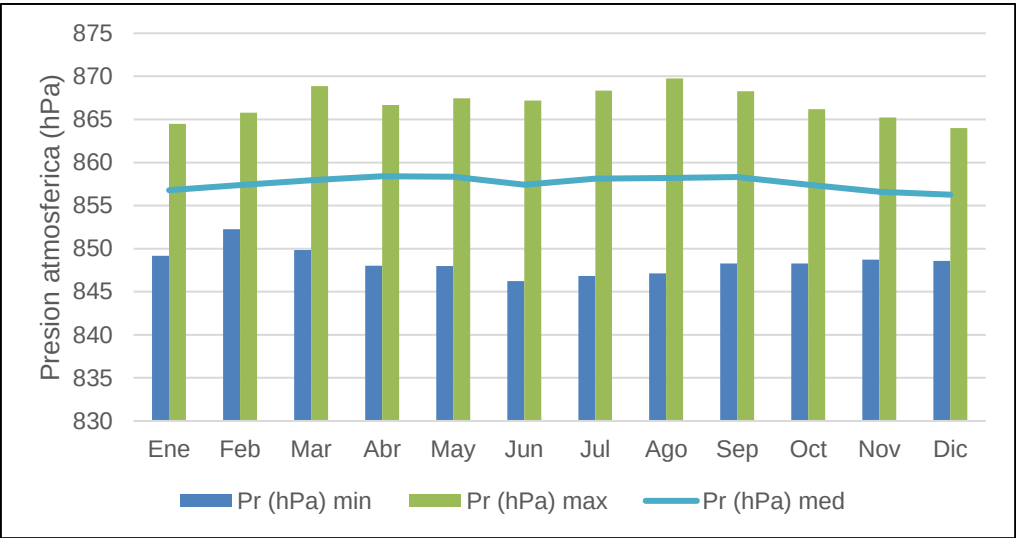
Gráfica 5.9 Presión atmosférica media mensual histórica 1993 a 2023
