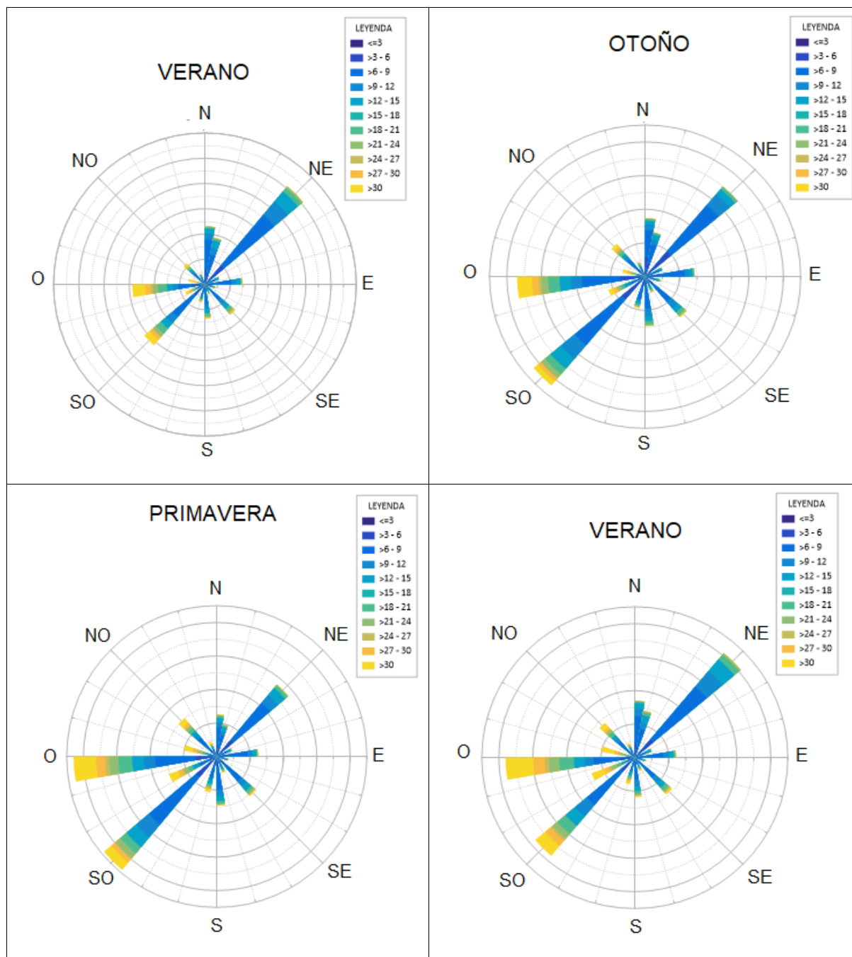
Gráfica 5.4 Rosa de los vientos por estación del período 1993-2023
