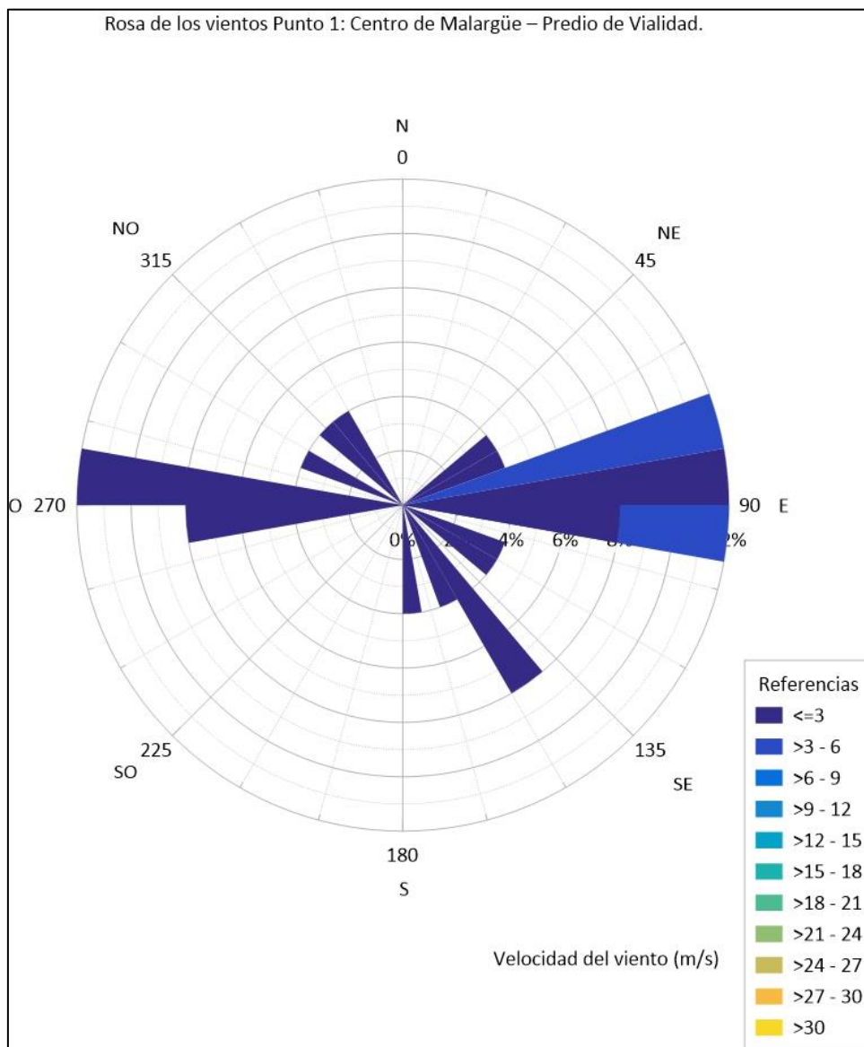
Figura 6.1 Rosa de los vientos durante el periodo de monitoreo. Punto 1: Centro de Malargüe – Predio de Vialidad
