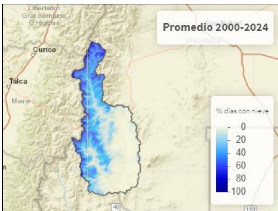
Figura 5.1 Porcentaje de días con nieve en la Cuenca del Río Colorado
