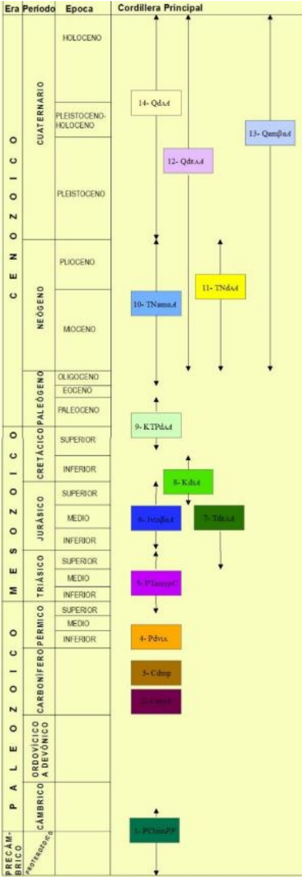
Figura 3.1 Referencia de las unidades tectonoestratigráficas
