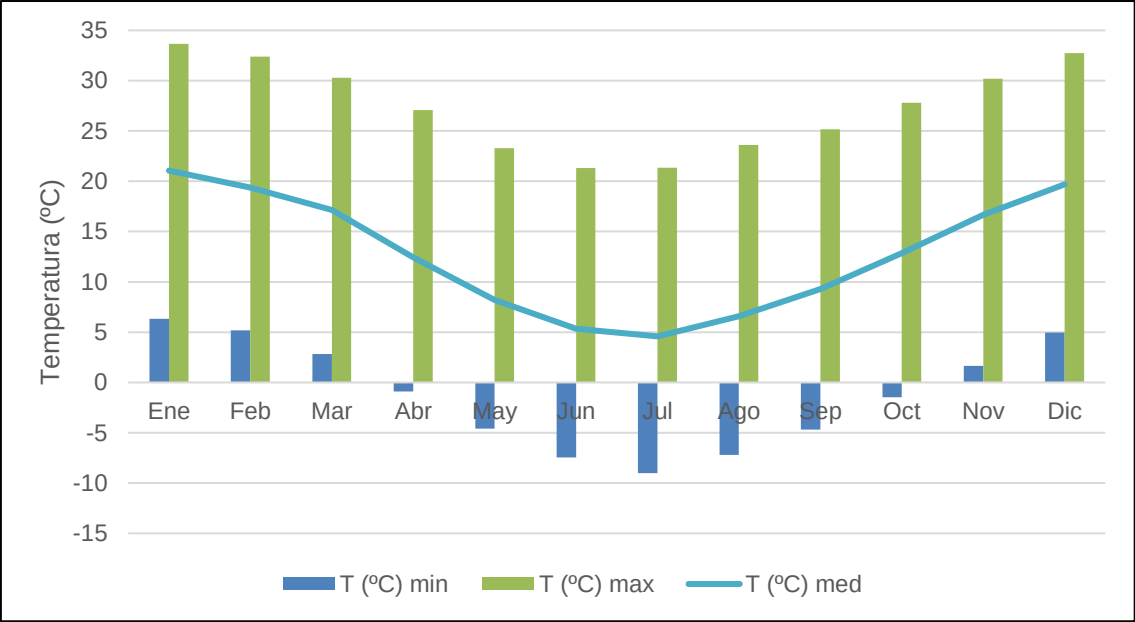
Gráfica 5.11 Temperatura de suelo media mensual del período 1993-2023
