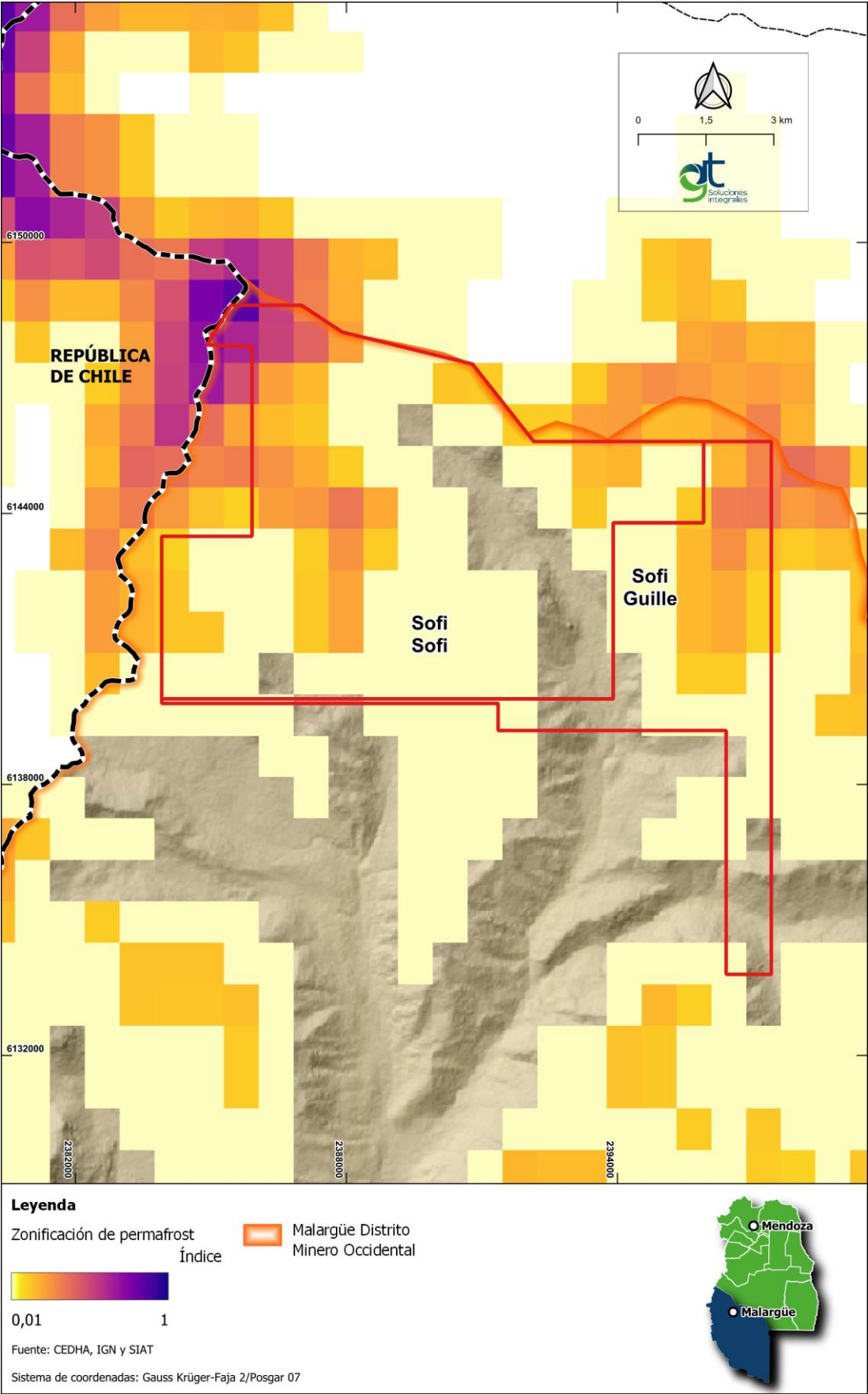
Mapa 4.2 Áreas de probabilidad de Permafrost
