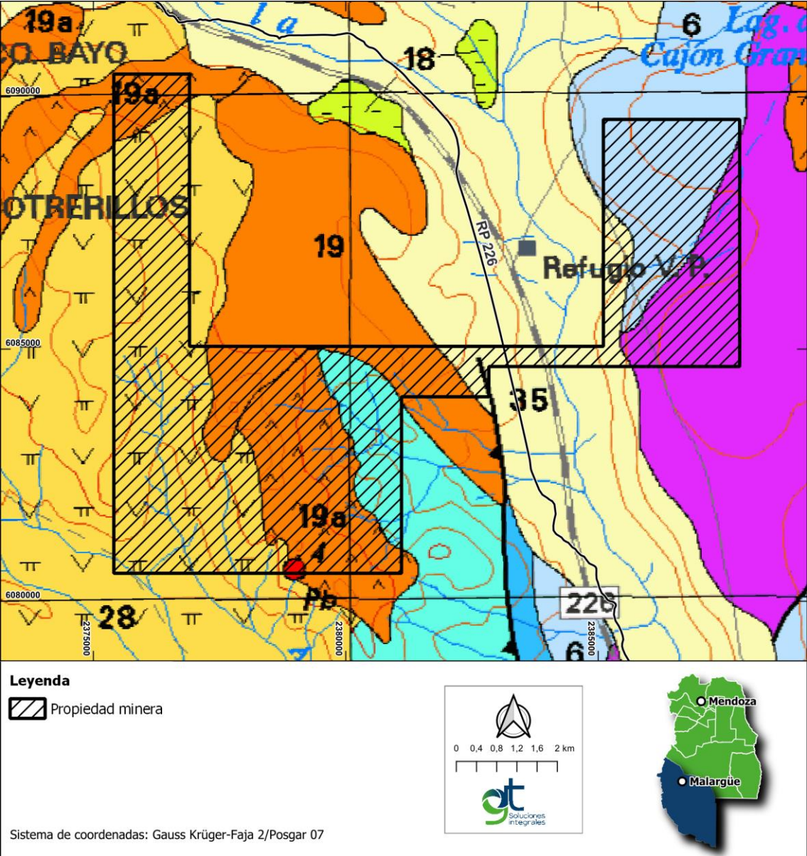
Mapa 3.1 Unidades geológicas aflorantes en el área de Proyecto
