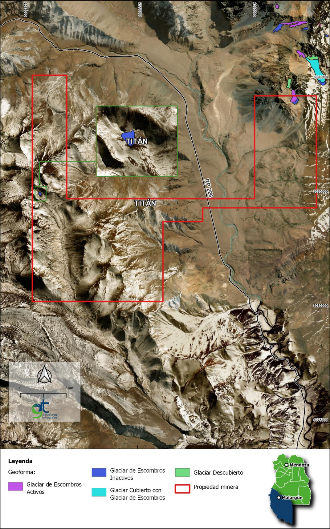
Mapa 4.1 Cuerpos Glaciares registrados en el área del proyecto
