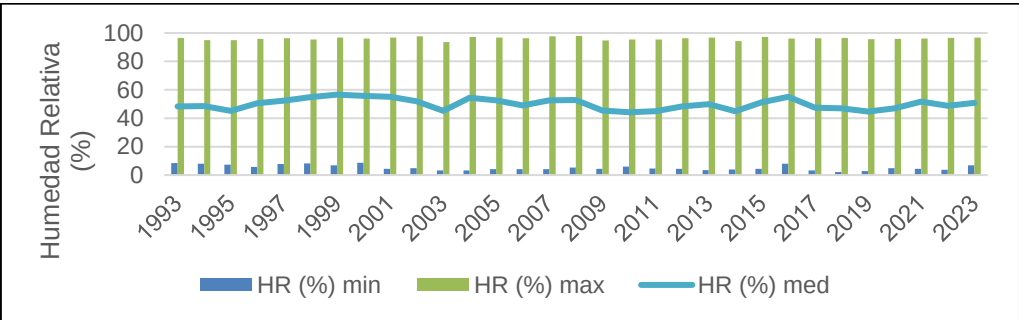
Gráfica 5.8 Humedad relativa anual del período 1993 a 2023
