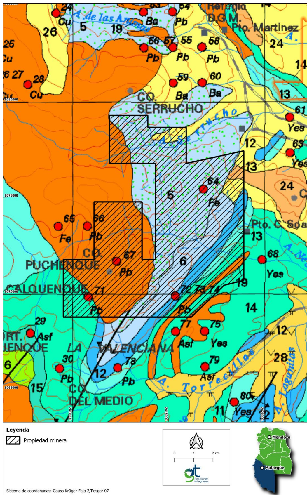
Mapa 3.1 Unidades geológicas aflorantes del área de Proyecto Tordillo
