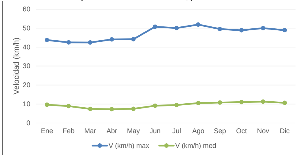
Gráfica 5.1 Velocidad promedio mensual del viento, período 1993-2023
