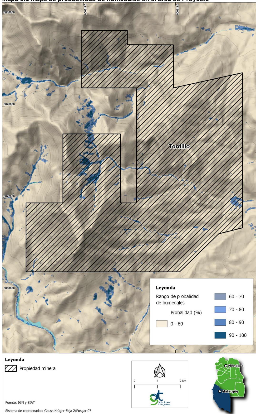
Mapa 9.1 Mapa de probabilidad de humedales en el área de Proyecto
