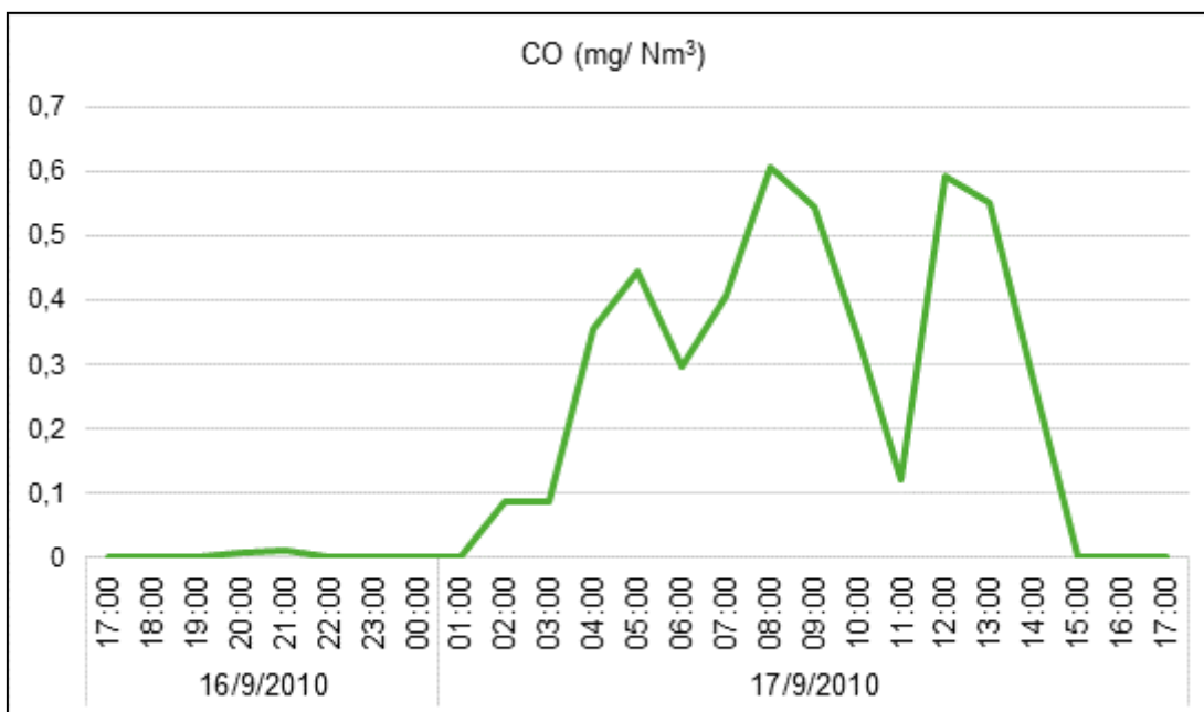
Gráfica 6.4 Variación de la concentración de CO durante el periodo de monitoreo. Punto 1: Centro de Malargüe – Predio de Vialidad
