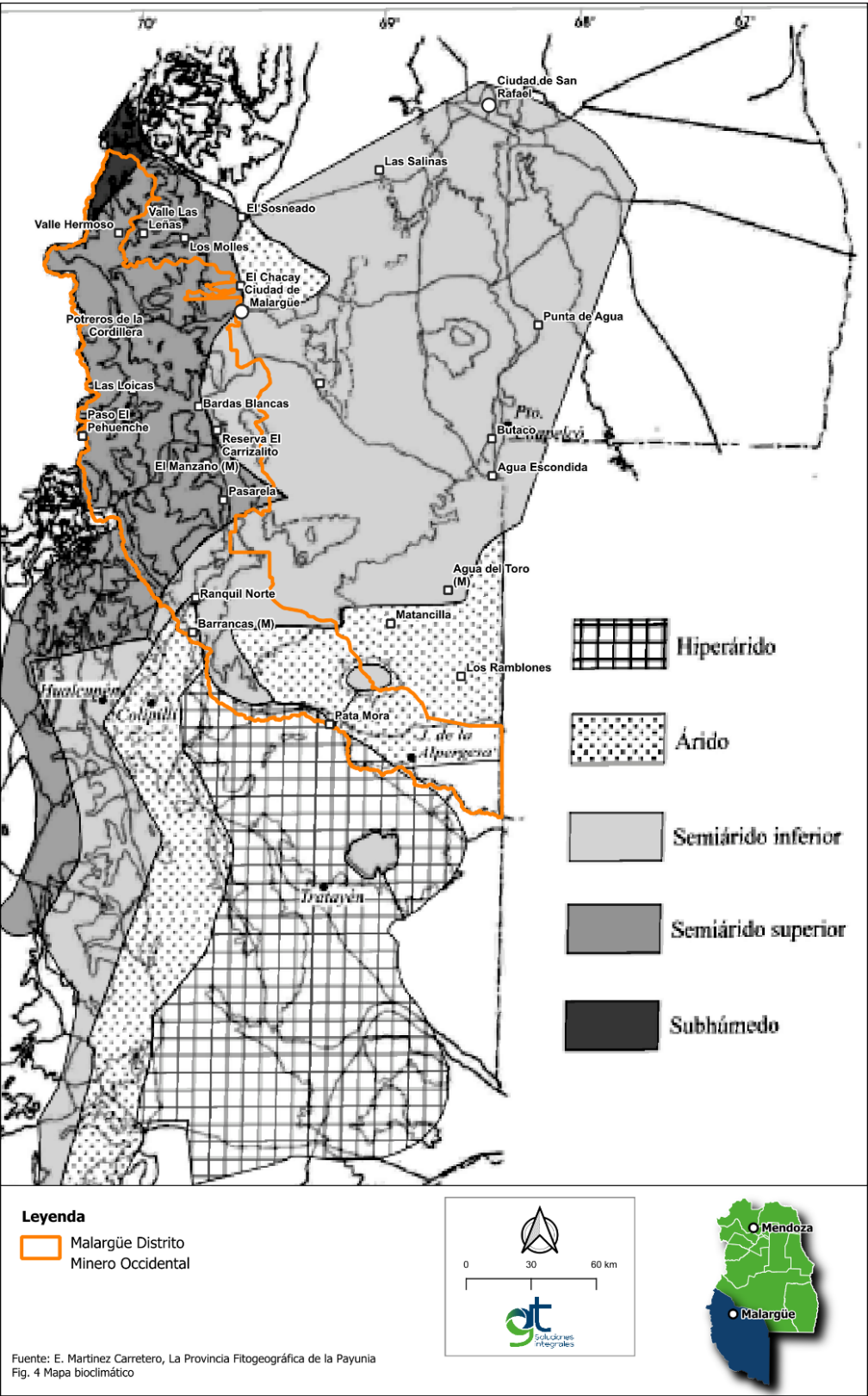
Mapa 5.1 Clasificación Bioclimática del Sur de Mendoza.
