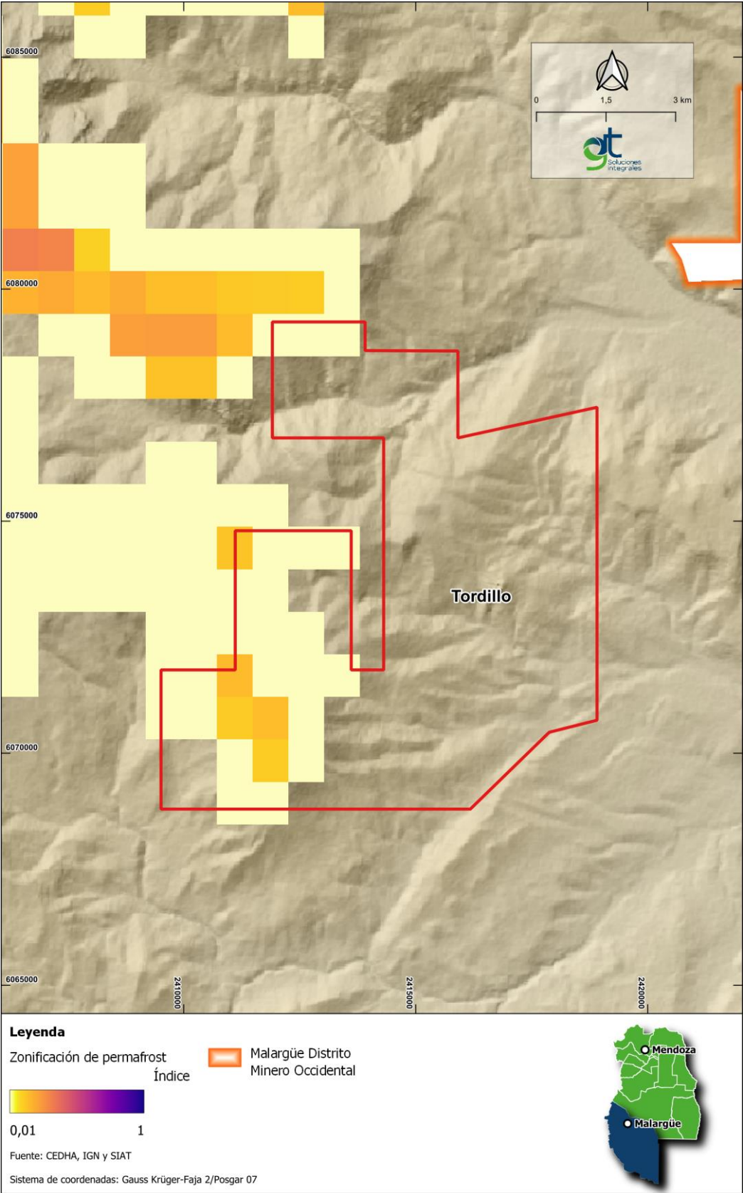
Mapa 4.2 Probabilidad de ambiente permafrost en el área de Proyecto
