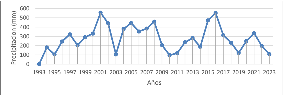
Gráfica 5.6 Precipitación acumulada anual del período 1993 a 2023
