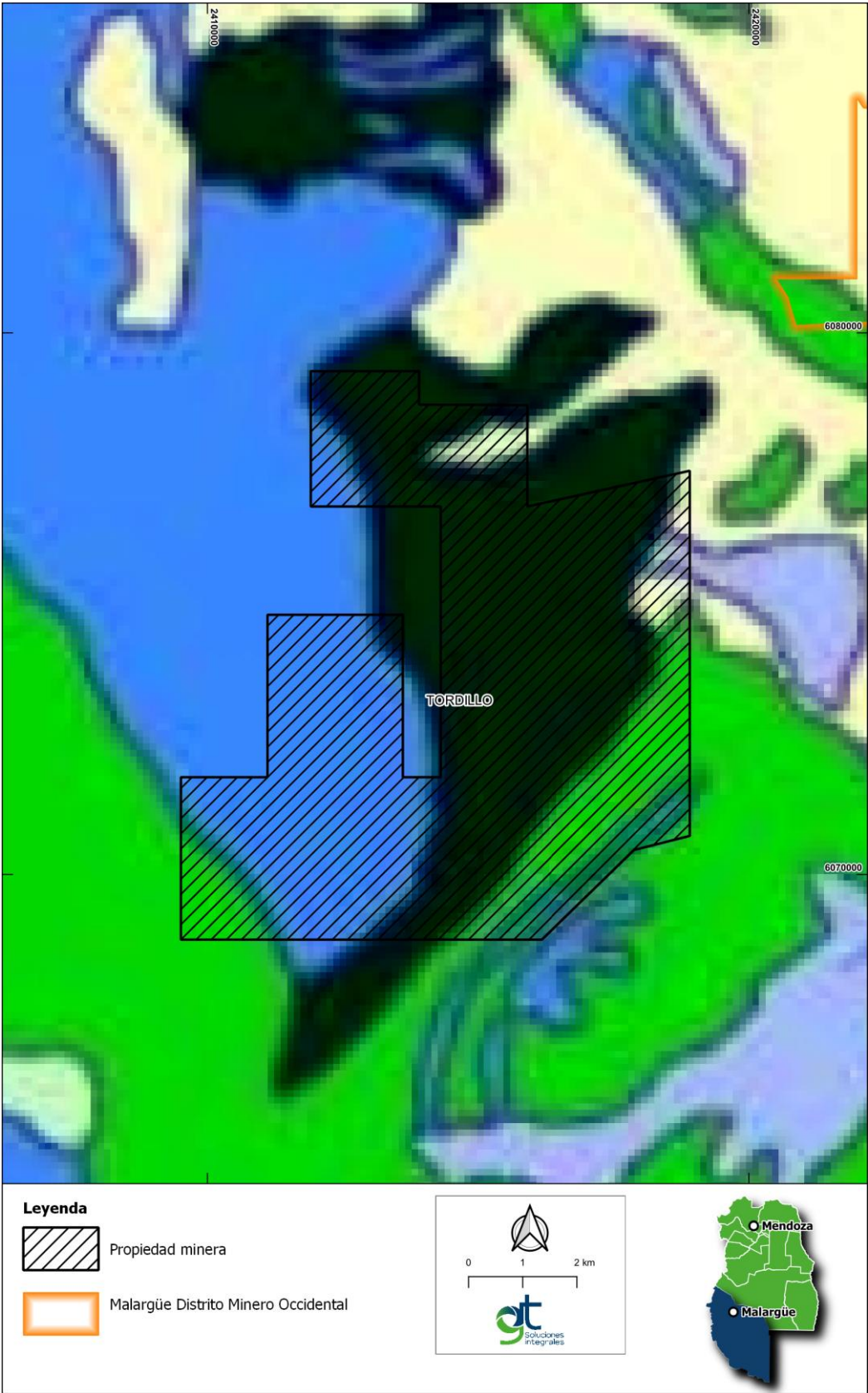
Mapa 3.2 Geología en el área de estudio
