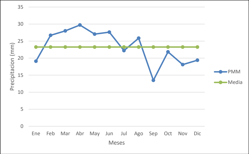
Gráfica 5.5 Precipitación media mensual del período 1993 a 2023
