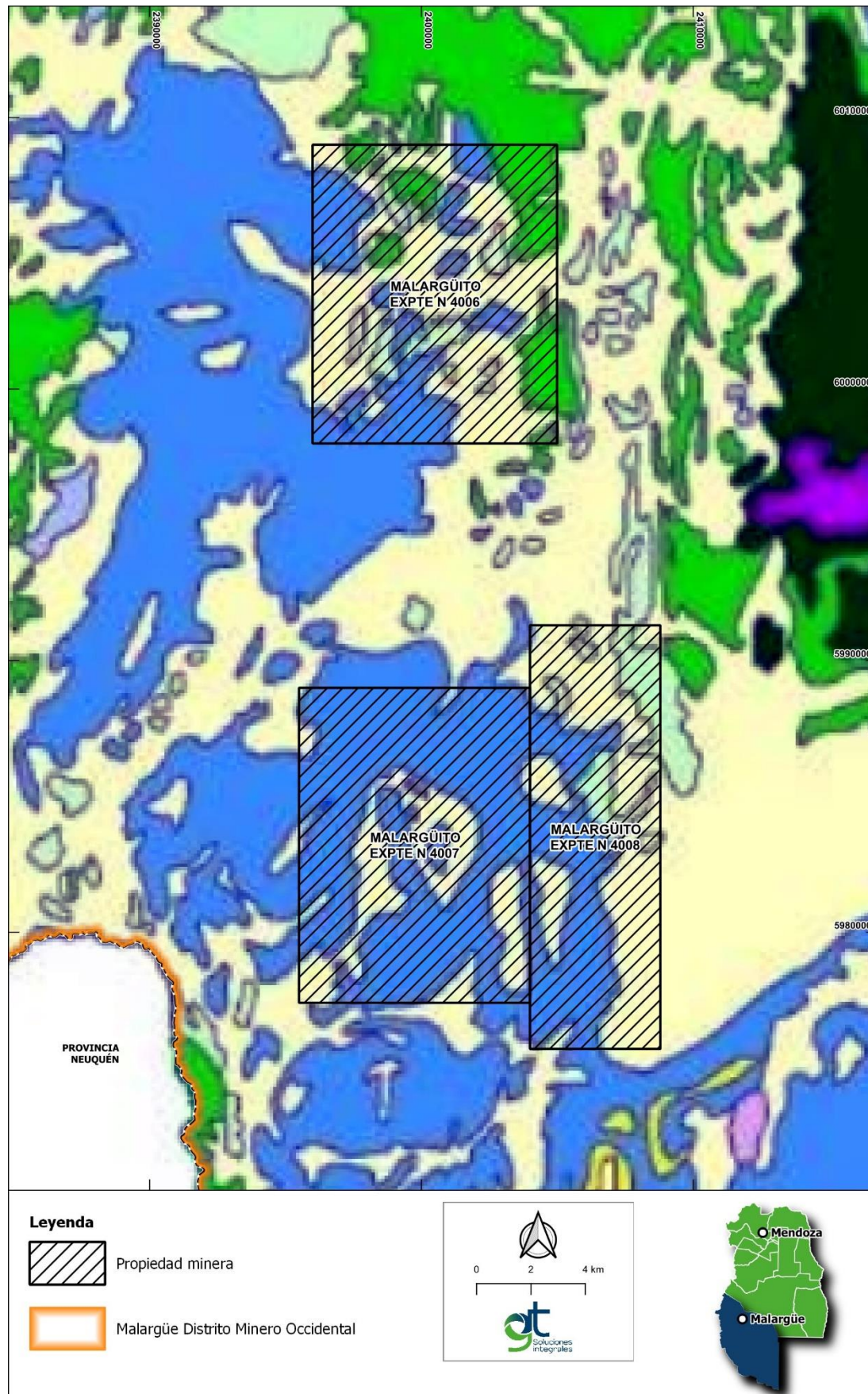
Mapa 3.2 Unidades tectonoestratigráficas del área de estudio
