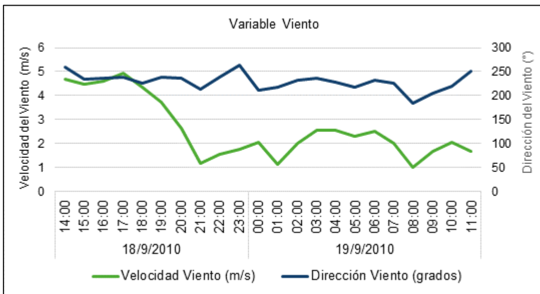
Gráfica 6.6 Variación de la velocidad y dirección del viento durante el periodo de monitoreo. Punto 4: Localidad Las Loicas – Puesto Vialidad.
