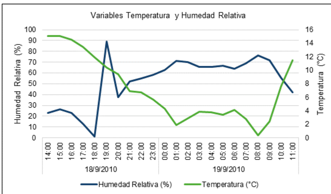
Gráfica 6.7 Variación de la temperatura y humedad relativa durante el periodo de monitoreo. Punto 4: Localidad Las Loicas – Puesto Vialidad
