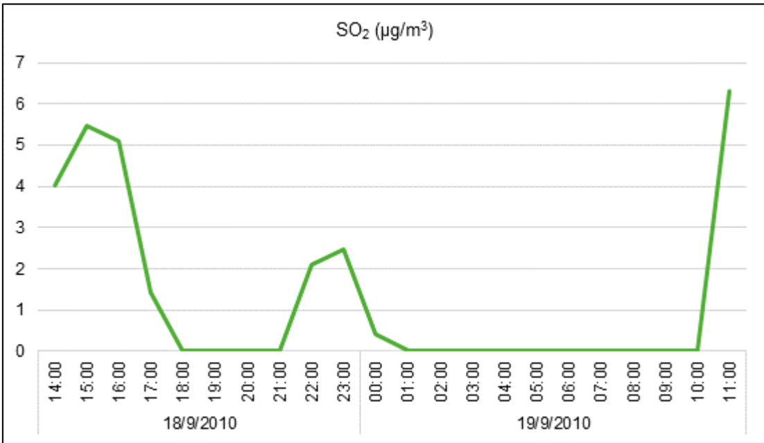
Gráfica 6.2 Variación de la concentración de SO 2 durante el periodo de monitoreo. Punto 4: Localidad Las Loicas – Puesto Vialidad
