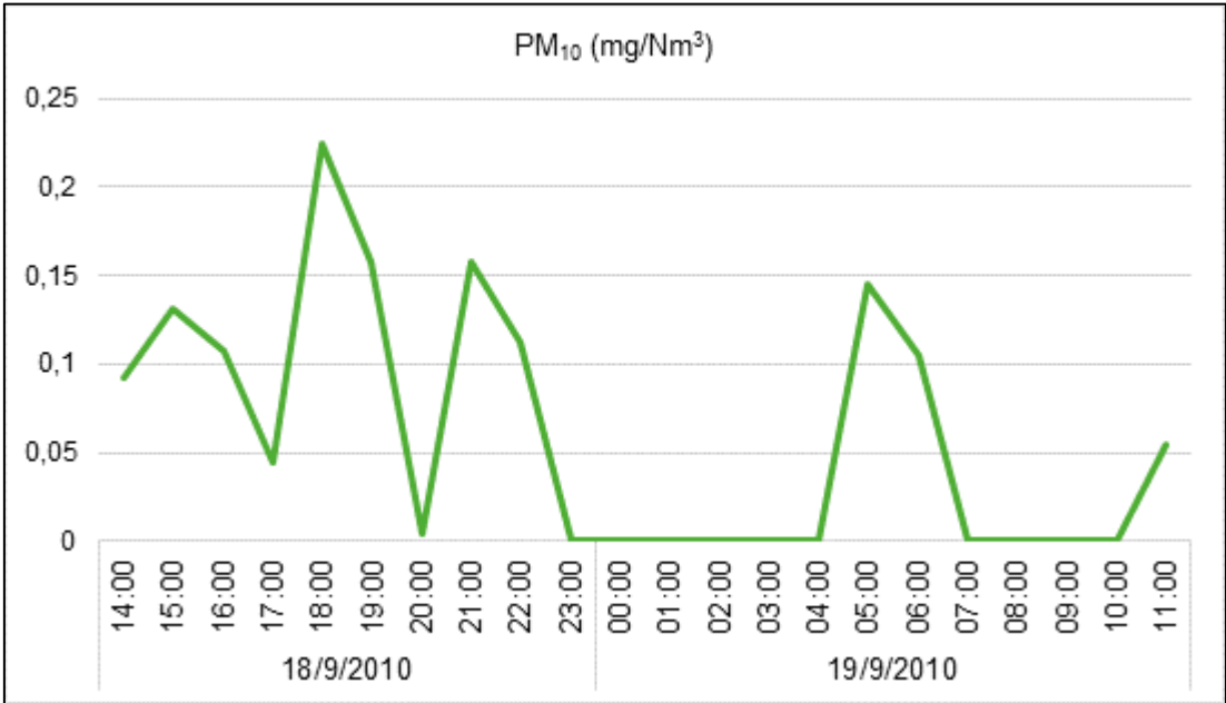
Gráfica 6.1 Variación de la concentración de PM 10 durante el periodo de monitoreo. Punto 4: Localidad Las Loicas – Puesto Vialidad
