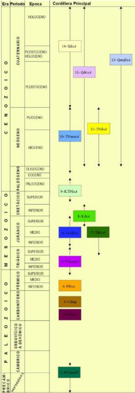
Figura 3.2 Referencia de las unidades geológicas
