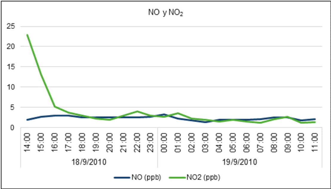
Gráfica 6.3 Variación de la concentración de NO yNO 2 durante el periodo de monitoreo. Punto 4: Localidad Las Loicas – Puesto Vialidad
