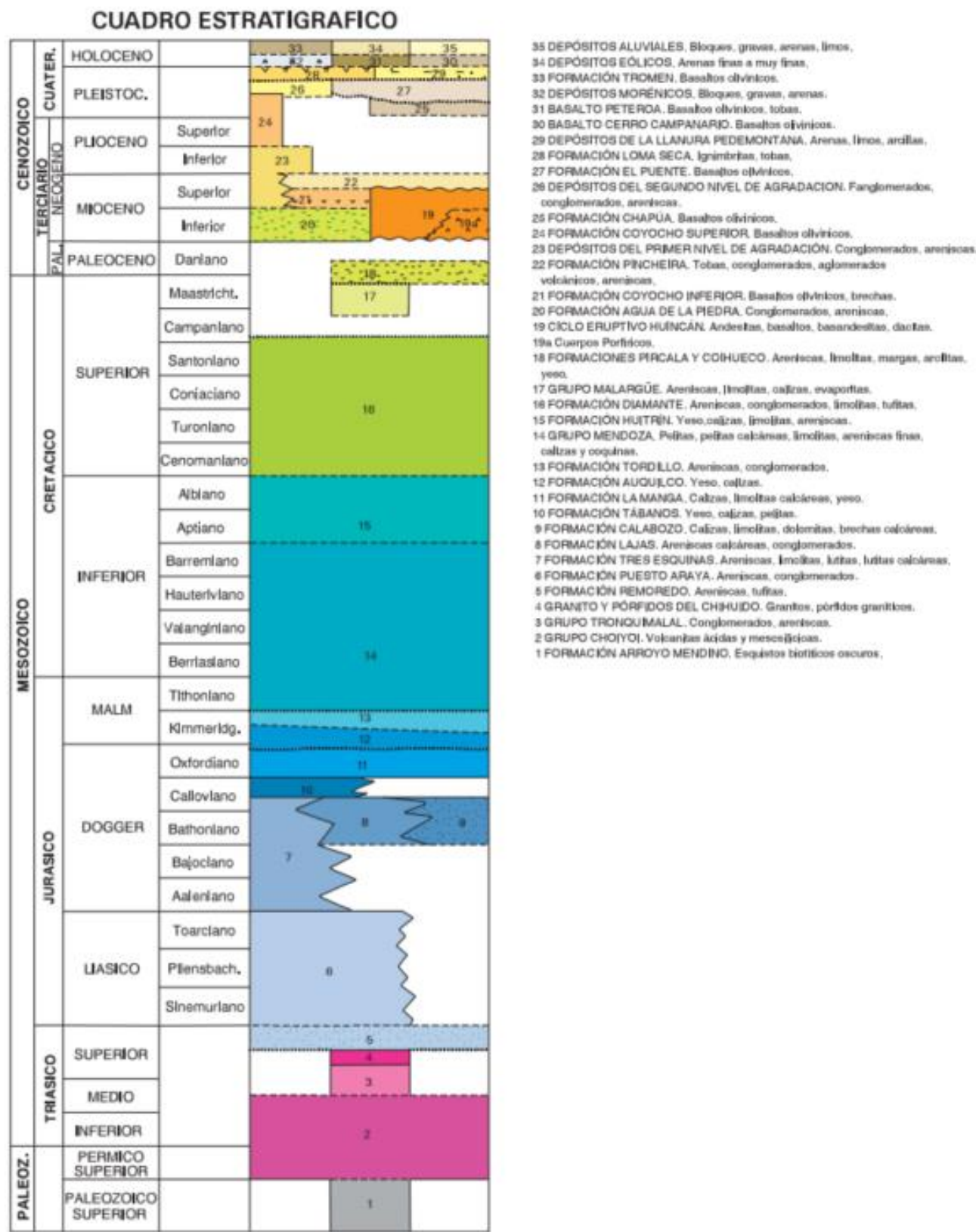
Figura 3.1 Referencias de la Hoja Geologica de Malargue (HG-3569-III)
