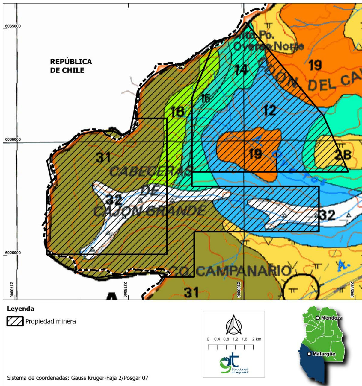
Mapa 3.1 Unidades geológicas aflorantes del área de Proyecto PAS
