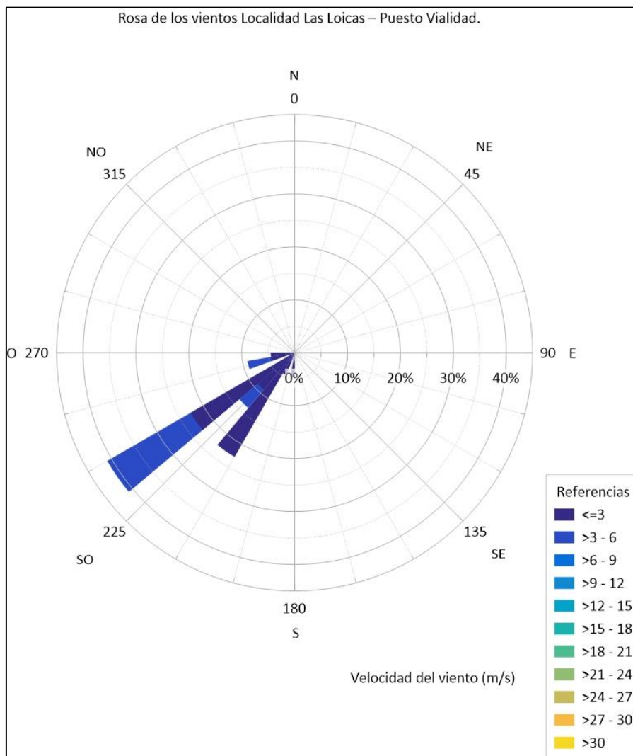
Figura 6.1 Rosa de los vientos durante el período de monitoreo. Punto 4: Localidad Las Loicas – Puesto Vialidad
