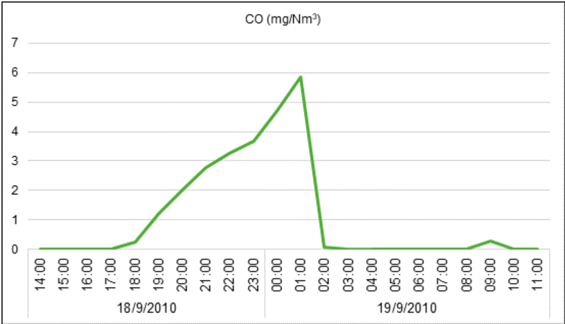
Gráfica 6.4 Variación de la concentración de CO durante el período de monitoreo. Punto 4: Localidad Las Loicas – Puesto Vialidad
