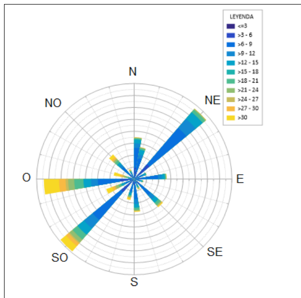
Gráfica 5.3 Rosa de los vientos promedio anual para el período 1993-2023
