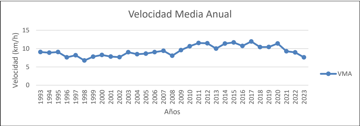
Gráfica 5.2 Velocidad del viento promedio anual período 1993-2023
