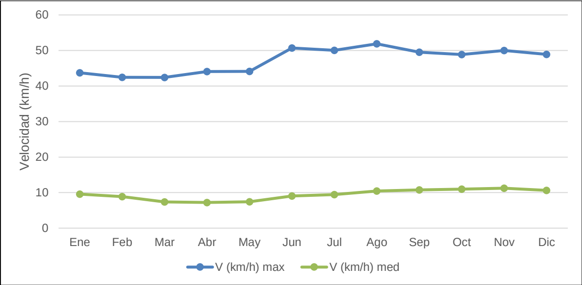
Gráfica 5.1 Velocidad promedio mensual del viento, período 1993-2023
