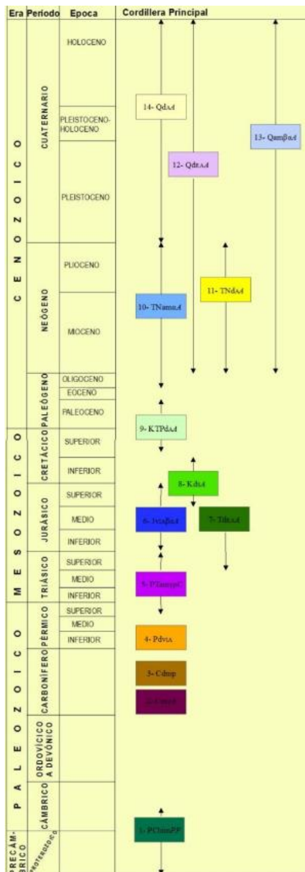
Figura 3.1 Referencia de las unidades tectonoestratigráficas
