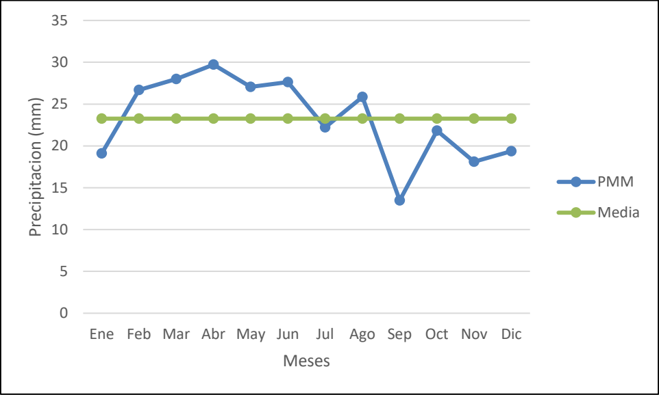
Gráfica 5.5 Precipitación media mensual del período 1993 a 2023
