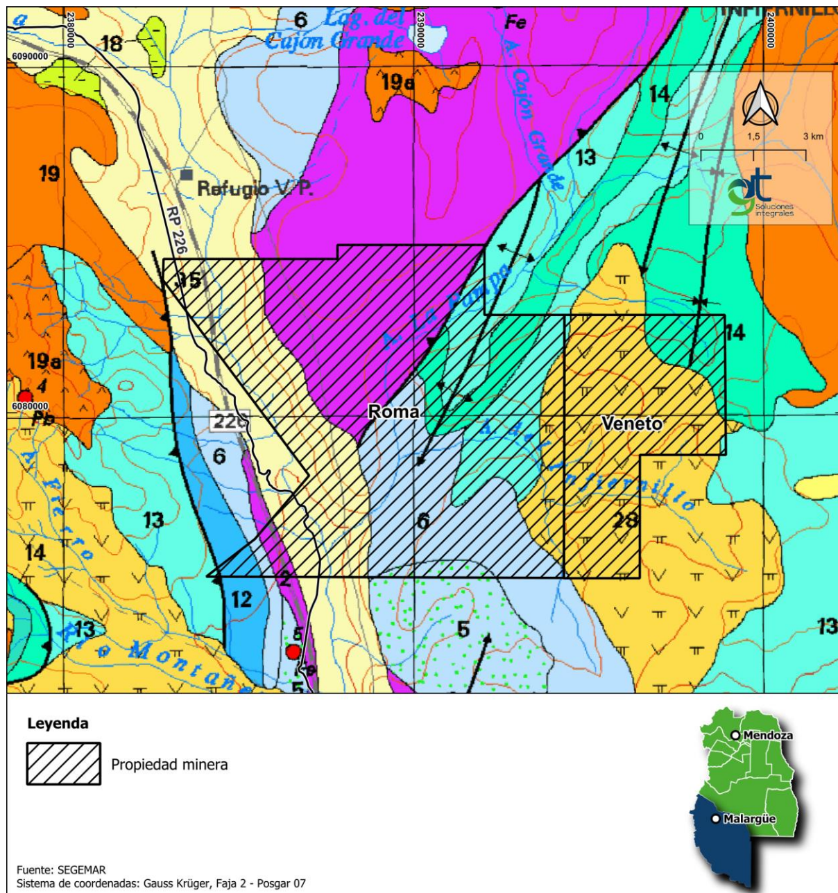
Mapa 3.1 Unidades geológicas aflorantes del área de Proyecto Roma y Veneto
