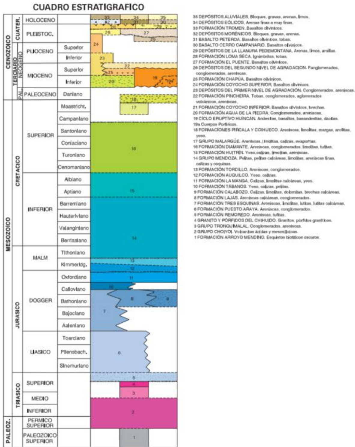
Figura 3.1 Referencias de la Hoja Geológica de Malargüe (HG-3569-III)
