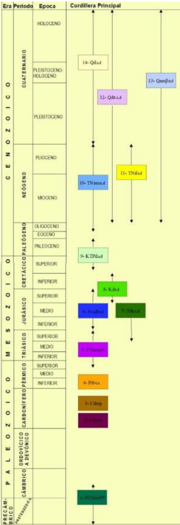
Figura 3.2 Referencia de las unidades geológicas
