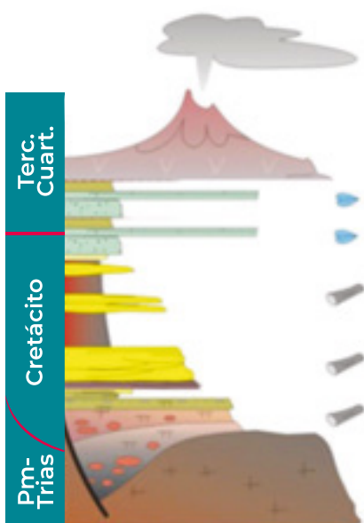
CUENCA NEUQUINA COLUMNA ESTRATIGRAFICA BORDE DE CUENCA
