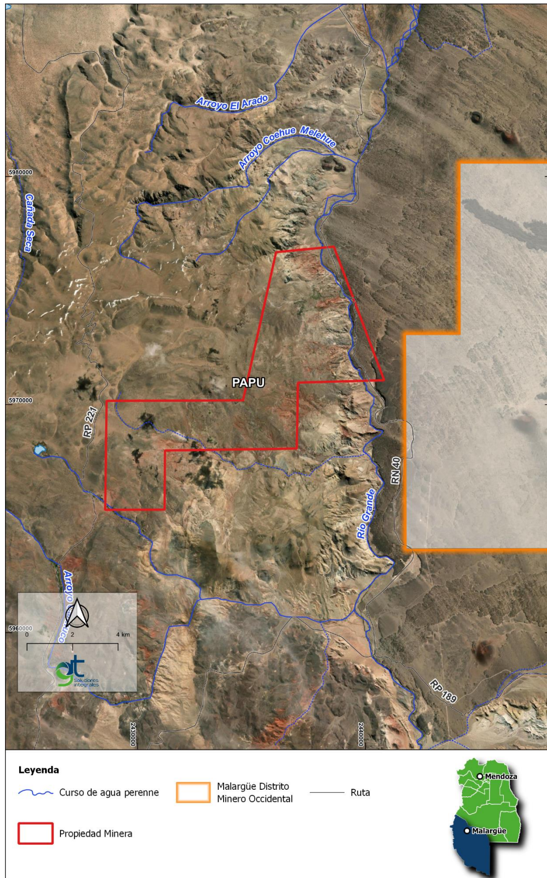
Mapa 7.1 Cursos y cuerpos de agua presentes en el área de Proyecto Papu.
