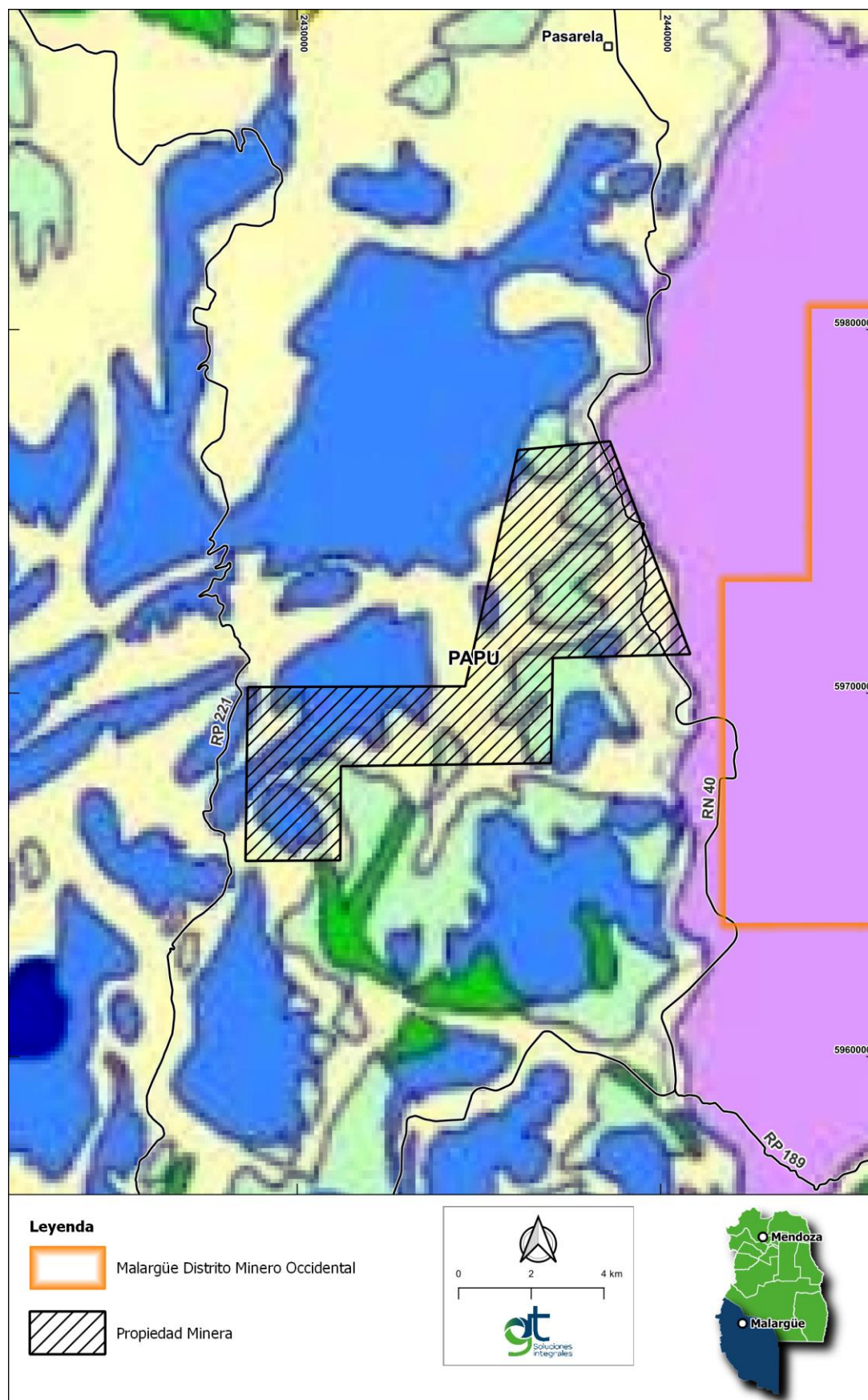
Mapa 3.1 Geología del área de Proyecto
