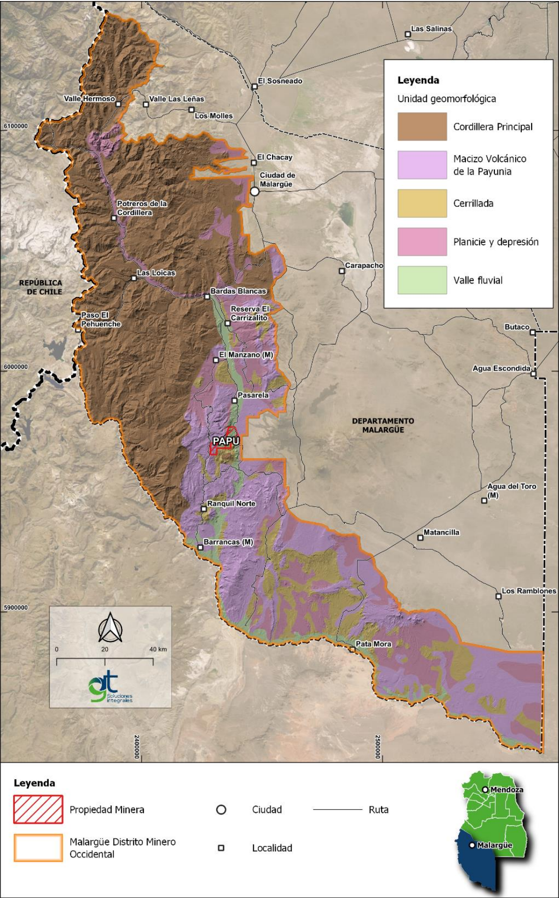
Mapa 3.2 Geomorfología del área de estudio
