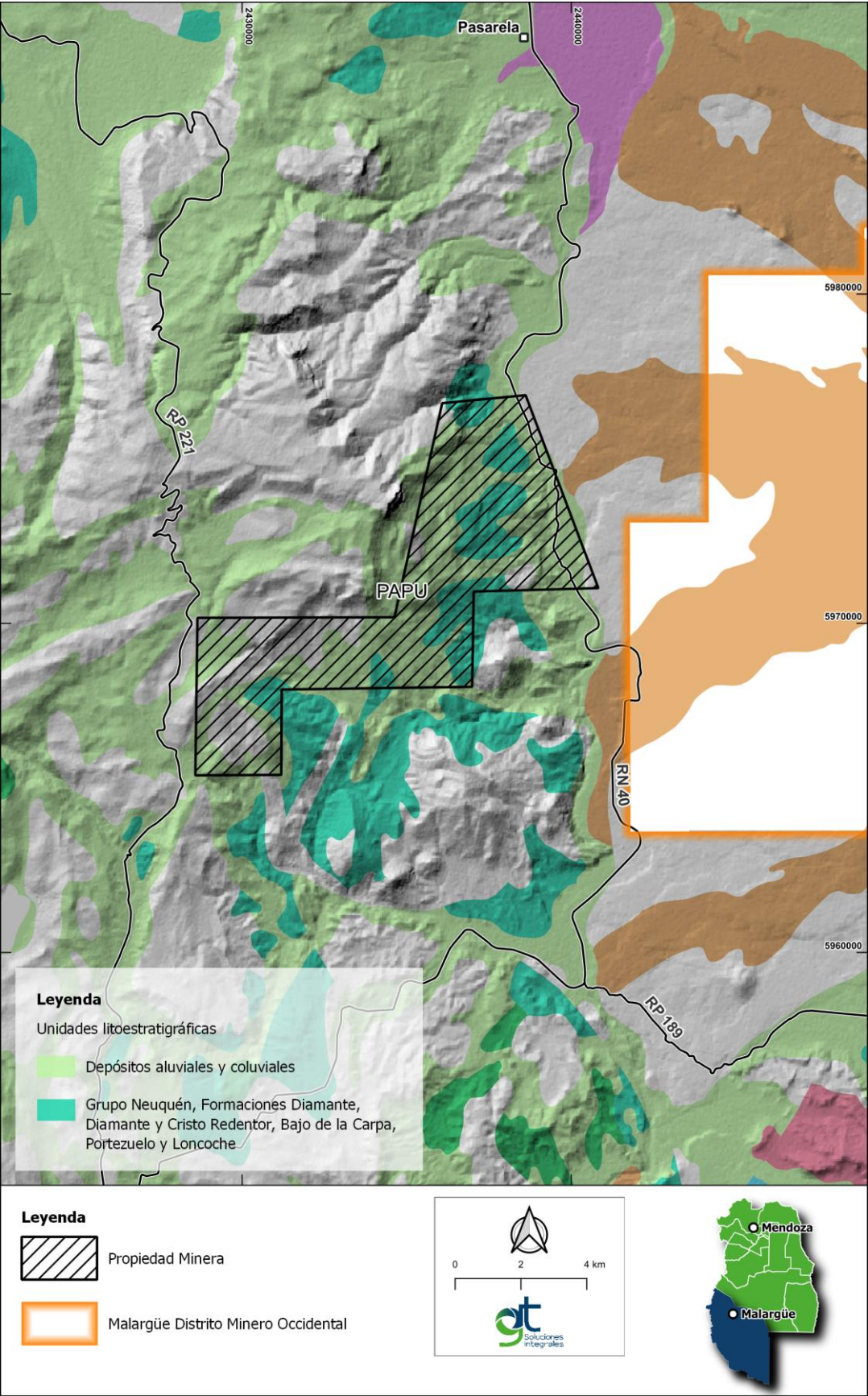
Mapa 15.1 Unidades litoestratigráficas
