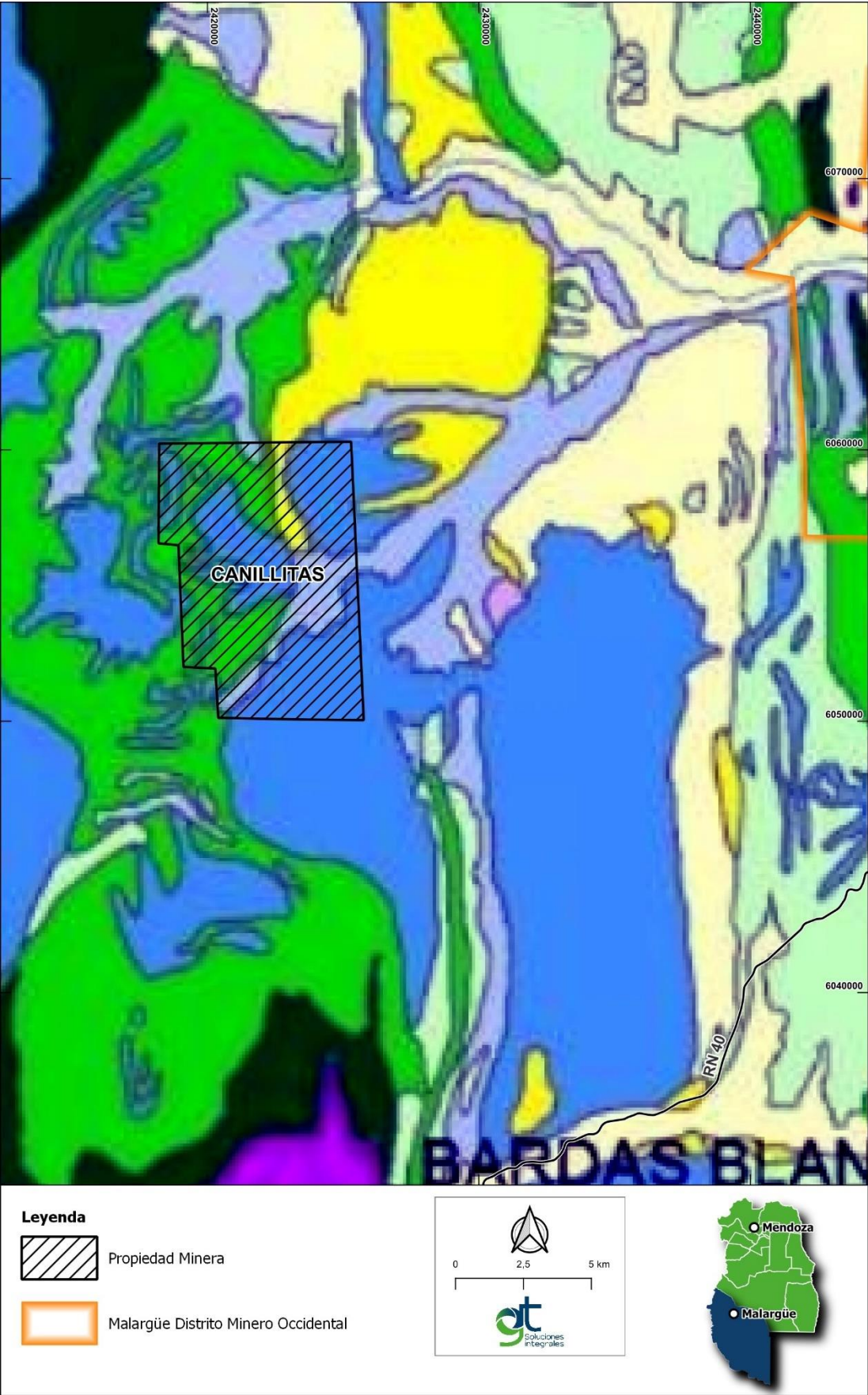
Mapa 3.1 Geología en el área de estudio
