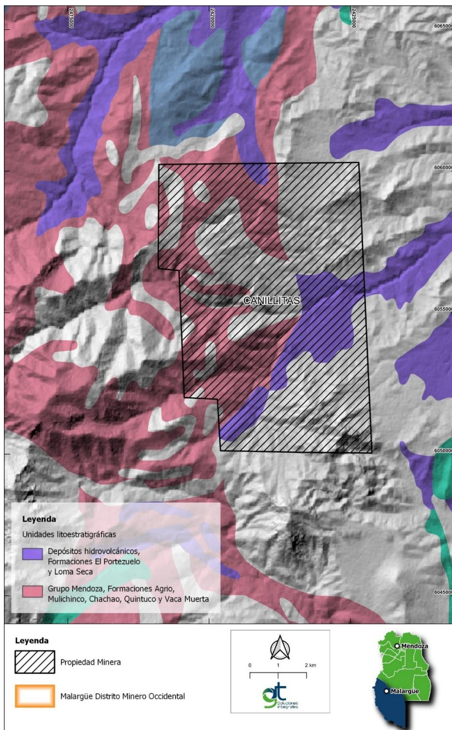
Mapa 15.1 Unidades litoestratigráficas
