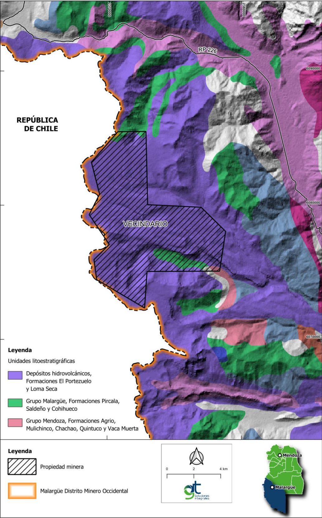
Mapa 15.1 Unidades litoestratigráficas
