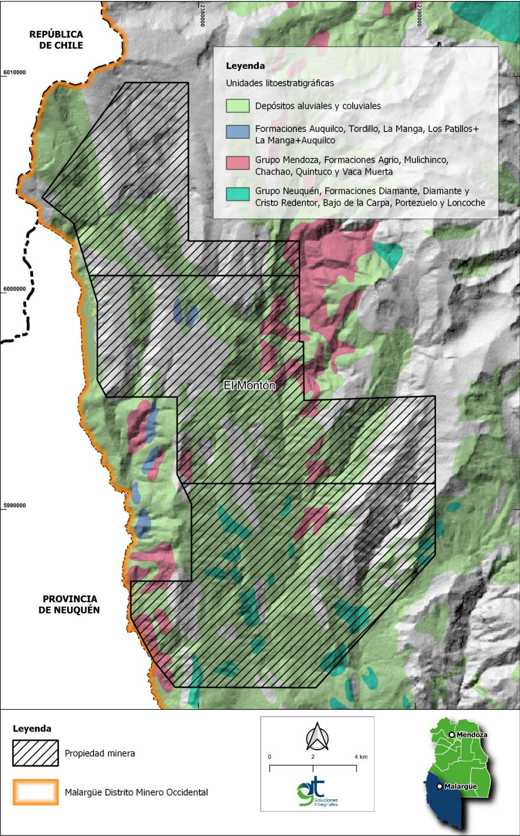
Mapa 15.1 Unidades Litoestratigráficas
